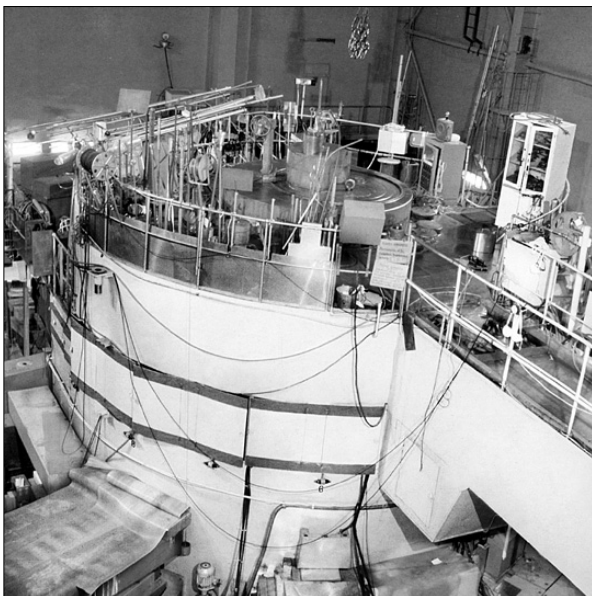
Дослідницький ядерний реактор ВВР-М, введений в експлуатацію в 1960. Київ.
