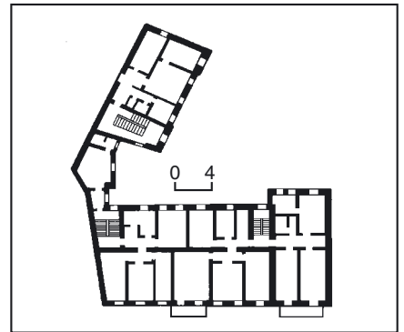
502.2. Вул. Софійська, 10. 502.2. План другого поверху.
