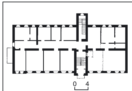
503.9. План першого поверху.
