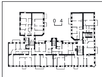
561.35. План другого поверху. 561.35. Вул. Червоноармійська, 43/16.
