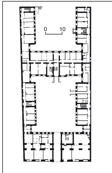
541.29. План першого поверху.
