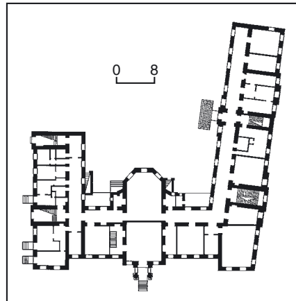
489.5.4. План першого поверху.
