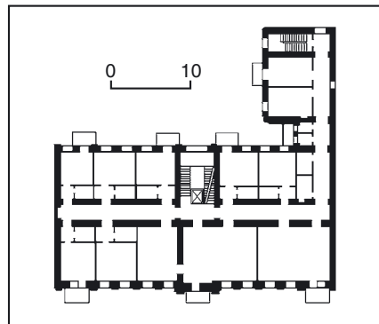
541.28. План другого поверху.
