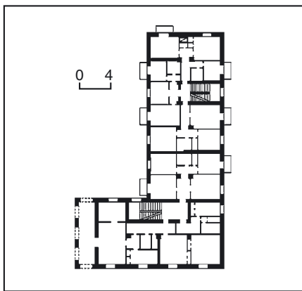
561.33. План третього поверху.
