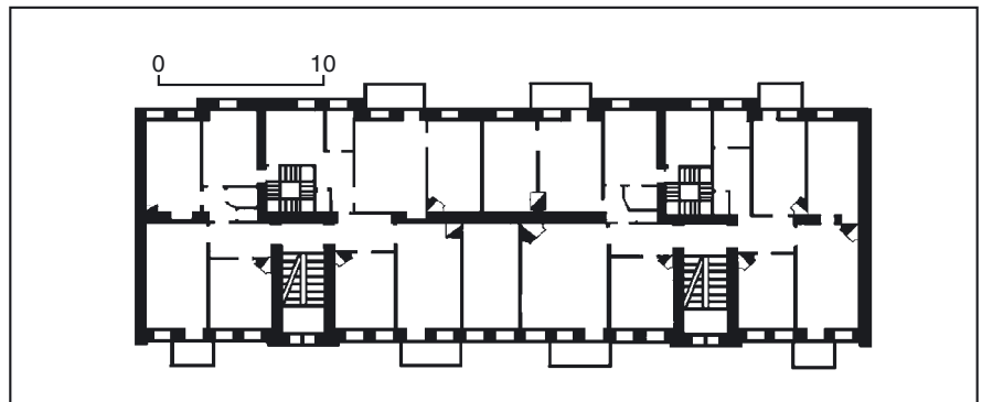
559.7. План другого поверху. 559.7. Вул. Чапаєва, 8.
