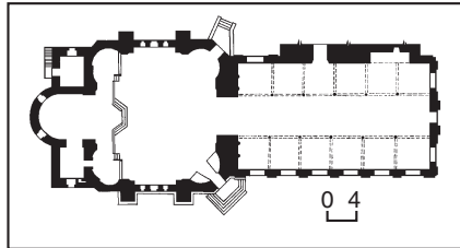
489.1.47. План першого поверху. 489.1.47. Трапезна палата з церквою в ім'я преподобних Антонія та Феодосія Печерських. Вигляд з північного заходу.
