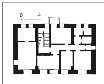
489.2.15. План першого поверху.
