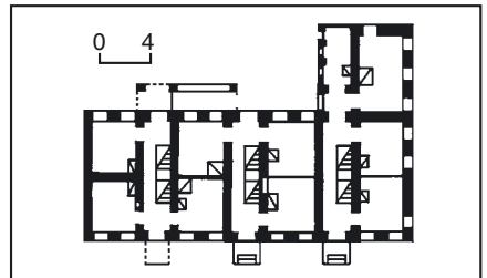
532.16. Келії. Корпус № 9. 532.16. План першого поверху.
