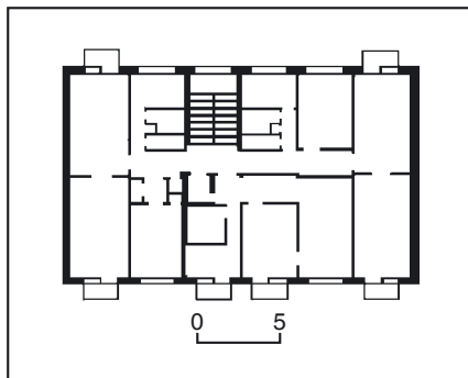
561.5. Вул. Червоноармійська, 16. 561.5. План третього поверху.
