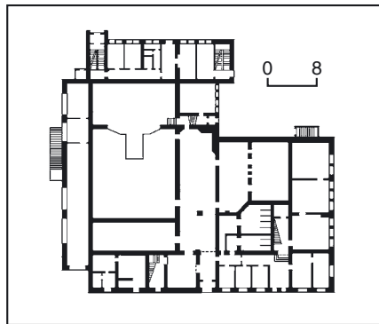
491. План першого поверху. 491. Просп. Голосіївський, 22.
