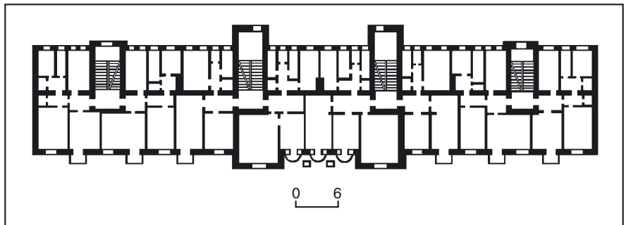
534.4. План четвертого поверху. 534.4. Вул. І. Франка, 9.
