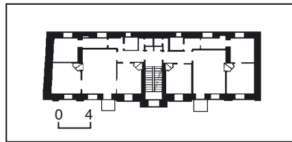
559.8. Вул. Чапаєва, 12. 559.8. План другого поверху.
