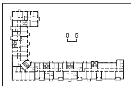
561.23. План першого поверху.
