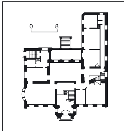
571.14. План першого поверху.
