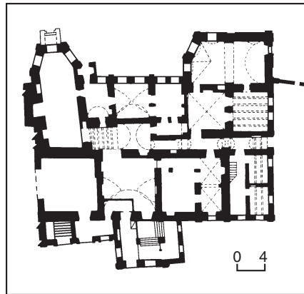
489.1.9. План першого поверху.
