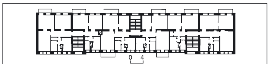
521.14. План другого поверху.
