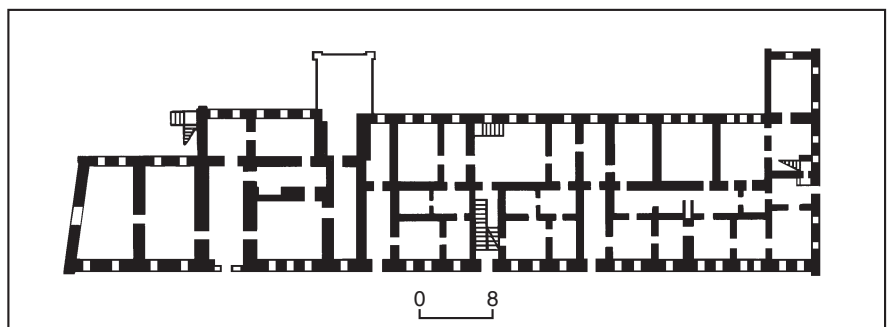
489.1.15. План першого поверху.
