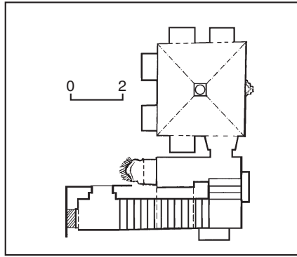
489.1.41. План споруди № 3.
