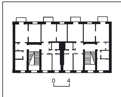
577.17. Вул. Ярославська, 30. 577.17. План другого поверху.
