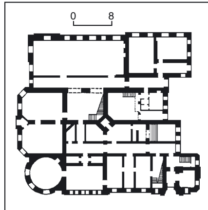
521.16. План першого поверху. 521.16. Вул. Л. Толстого, 7/2. Особняк.
