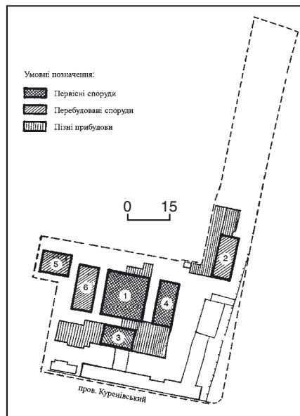
536. Генеральний план:
