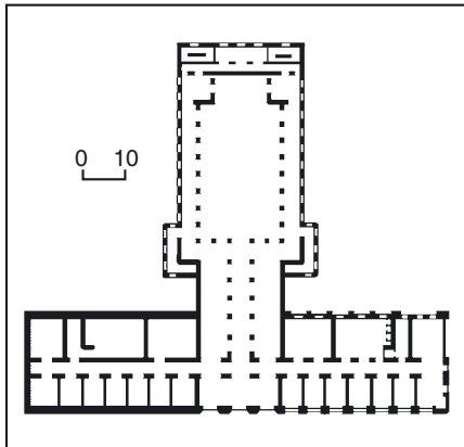
544.7. План третього поверху.
