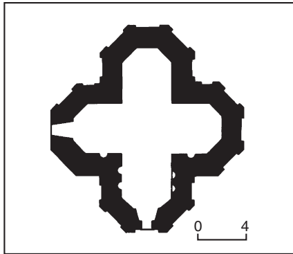
489.1.33.2. План першого ярусу.
