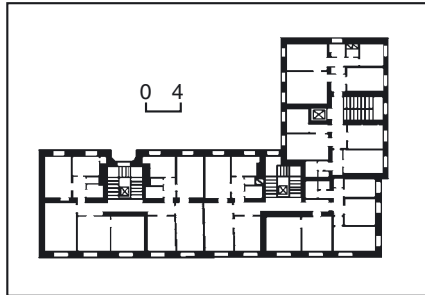
563.14. План другого поверху.
