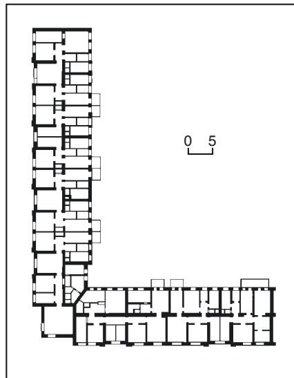
576.14. План Другого поверху.
