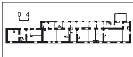
532.13. План першого поверху. 532.13. Келії. Корпус № 6.
