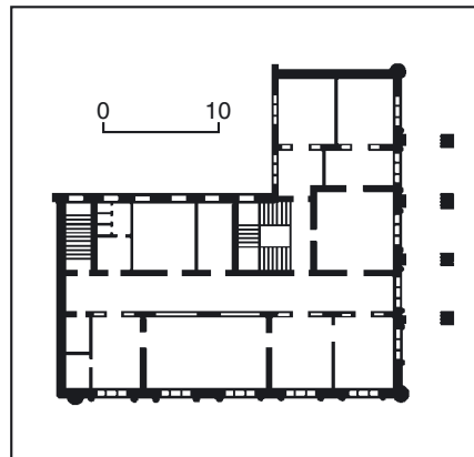
544.6. План третього поверху.
