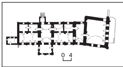
489.1.40. План.
