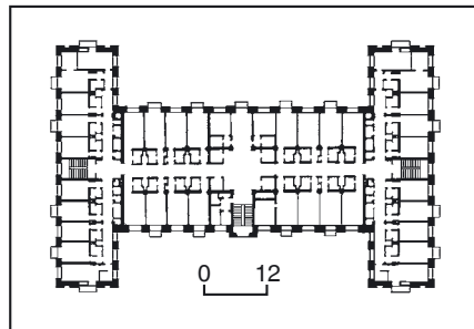
544.1.2. План п'ятого поверху.
