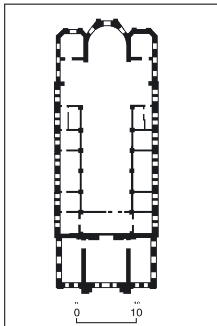
494. Вул. Ш. Руставелі, 13. 494. План другого поверху.
