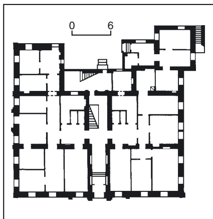
534.11. План першого поверху.
