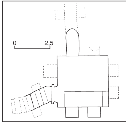
489.1.41. План споруди № 35.
