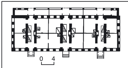
532.17. План першого поверху. 532.17. Келії. Корпус № 10.
