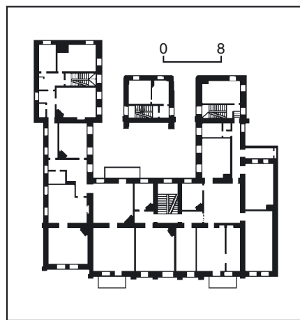
534.13. План другого поверху.
