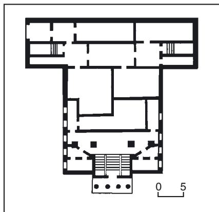
309.5. План першого поверху.
