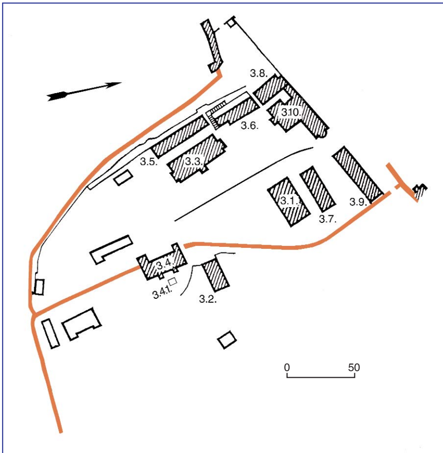
489.3. Гостиний двір. Генеральний план.
