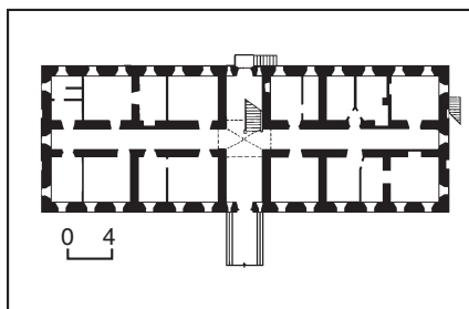
489.3.5. План першого поверху.
