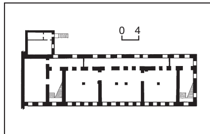
489.1.26. План другого поверху.
