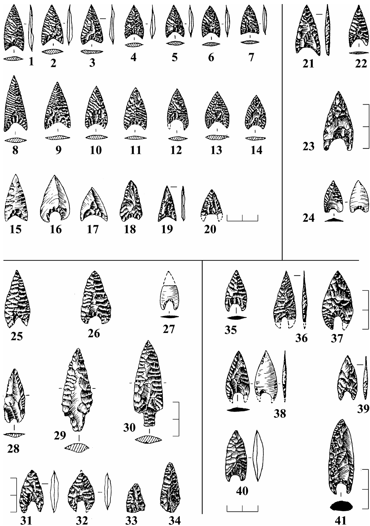
Рис. 60. Доба середньої бронзи. Культура багатоваликів кераміки. 1–7. Миколаївка 1.8; 8–14. Бєєва Могила 3; 15–17. Близьнюки 1.1; 18–20. Кременчук; 21. Нові Раскаєнці 1.15; 22. Прядівка 6.1.1; 23. Новопідкрязь 6.1.1; 24. Н. Бараніковка 5.10; 25–27. Бабино 3; 28–30. Шахта 22, 3.3; 31–34. Текстильник 2.5; 35. Кулішівка 425.56; 36. Керчік 17.9; 37. Миколаївка; 38. Молодогвардійськ 2.5; 39. В. Знам'янка; 40. Новопідкрязь 4.15; 41. Новопідкрязь 5.1.1.
