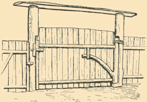
Мал. 10. Ворота на саморідному бігуні.
