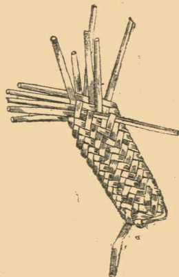
Рис. 49. Плетінка одинадцятикінцівка
