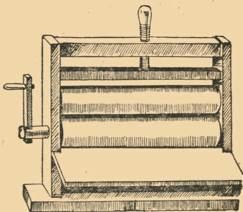
Рис. 9. Прес
