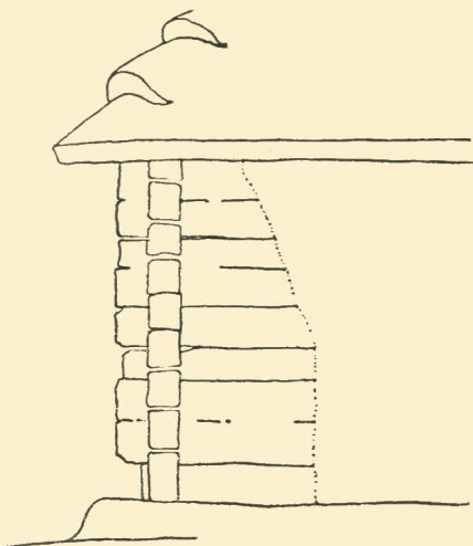
46. Рубка угла с одинаковыми остатками. Киевщина.
