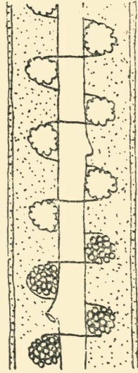
54. Заборка каркаса камышом и глиной. Полтавщина.
