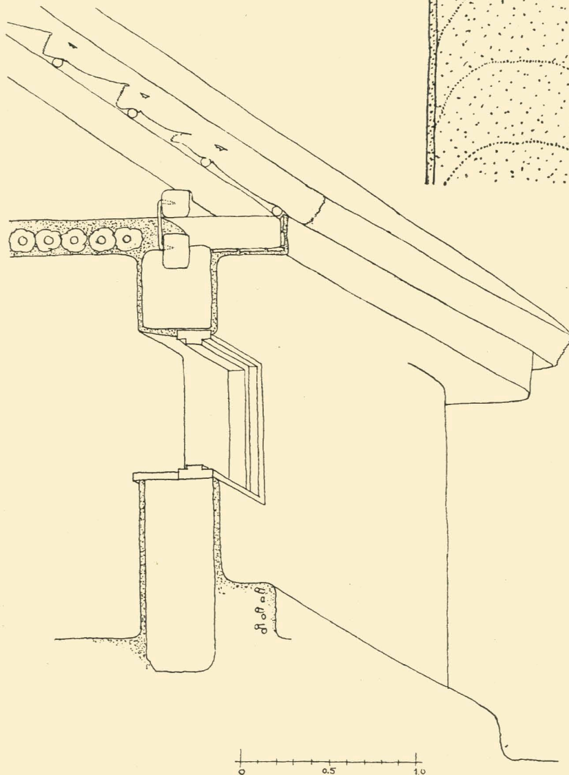
58. Конструкция хаты при глиняных стенах. Киещина.
