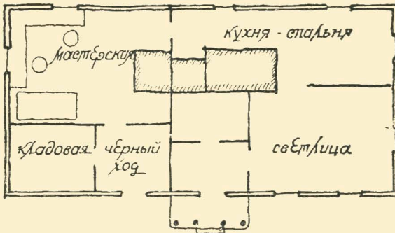
42. Хата гончара. Село Опожня. Полтавщина (по М. Русову).
