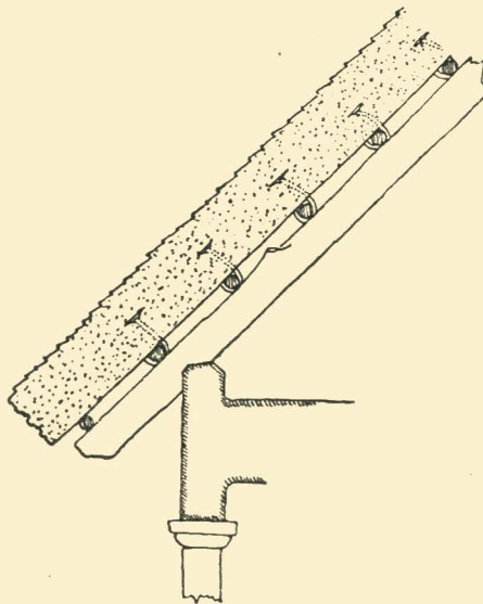
70. Конструкция кровли из камыша. Полтавщина.
