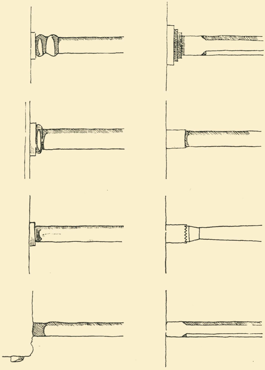
85. Обработка верха столов. Полтавщина, Подольщина, Киевщина.
