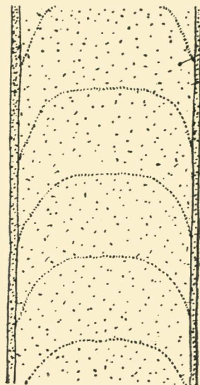
57. Конструкция стены из глиняных вальков. Киещина.
