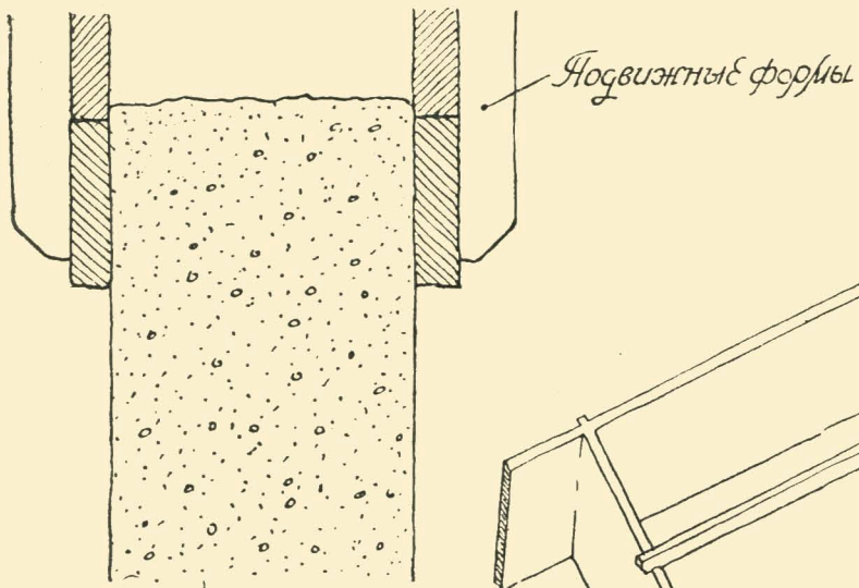
59. Глинобитная стена с подвижной формой. Днепропетровщина.
