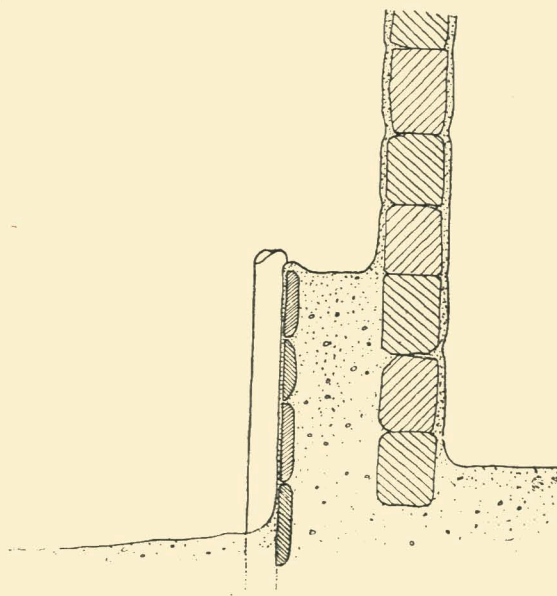
48. Конструкция „призвби“. Полтавщина.
