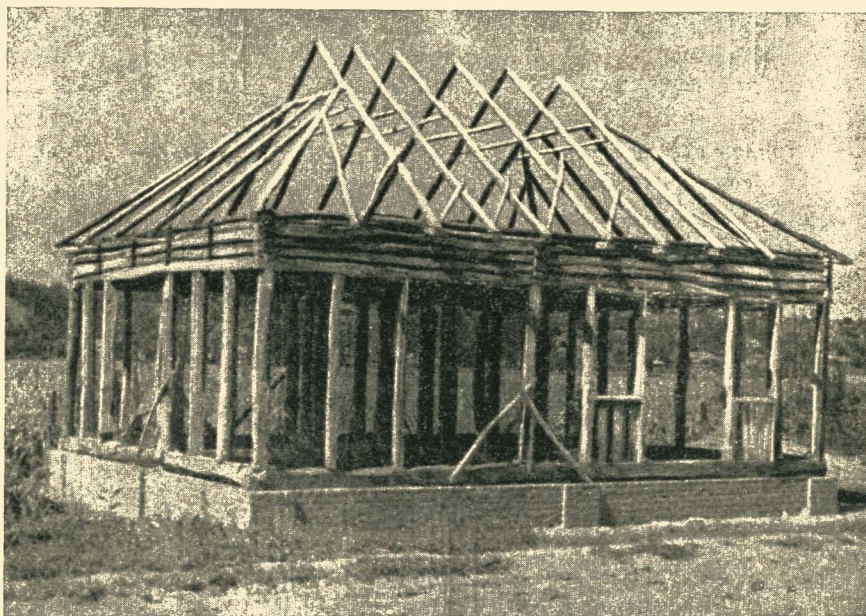
49. Конструктивный скелет каркасной хаты. Село Засулье. Полтавщина.
