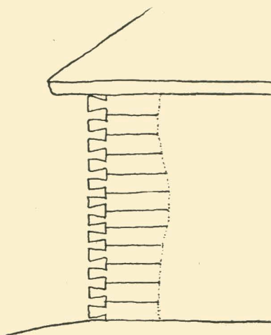
47. Рубка угла в лапу. Полесье.
