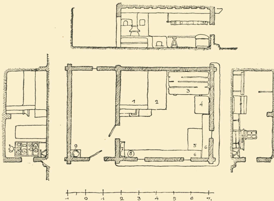
26. Типичная внутренняя организация однокомнатной хаты. План и разрезы. Село Медвин. Киевщина.
