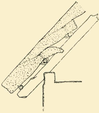
66. Конструкция свеса соломенной кровли.
