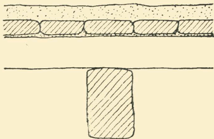
61. Конструкция потолка с главной и второстепенными балками. Киевщина.
