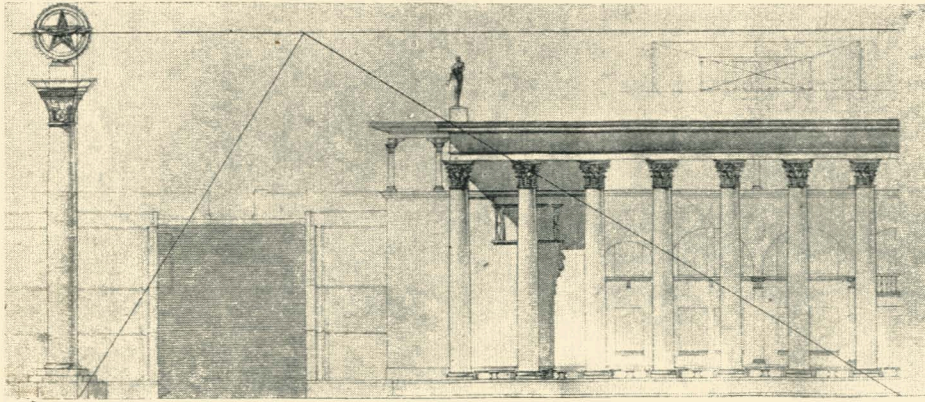
Побудова основних пропорцій головного фасаду спортивного павільйону.
