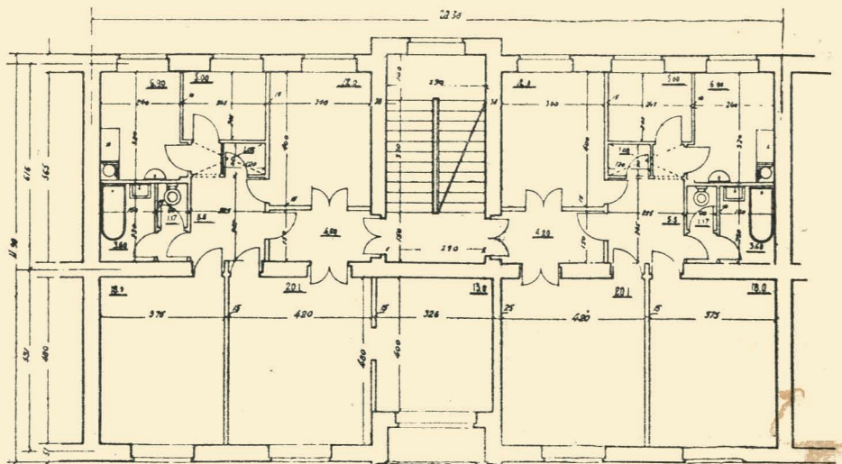
Архіт. Л. Киселевич і І. Хоменко (під керівн. архіт. М. Холостенка—Київ). Проект 3,5 і 4,5 кімнатної квартири. Жила площа 4,5-кімн. квартири—68 м 2 , k_1 = 0,74 . Жила площа 3,5-кімн. квартири 55 м 2 , k_1 = 0,70 .
