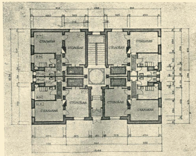
Архіт. Заславський (Київ). Двокімнатна квартира в двоповерховому 8-квартирному будинку для села (без каналізації). Жила площа—32 м 2 , k_1 = 0,62 , k_2 = 8,8 .
