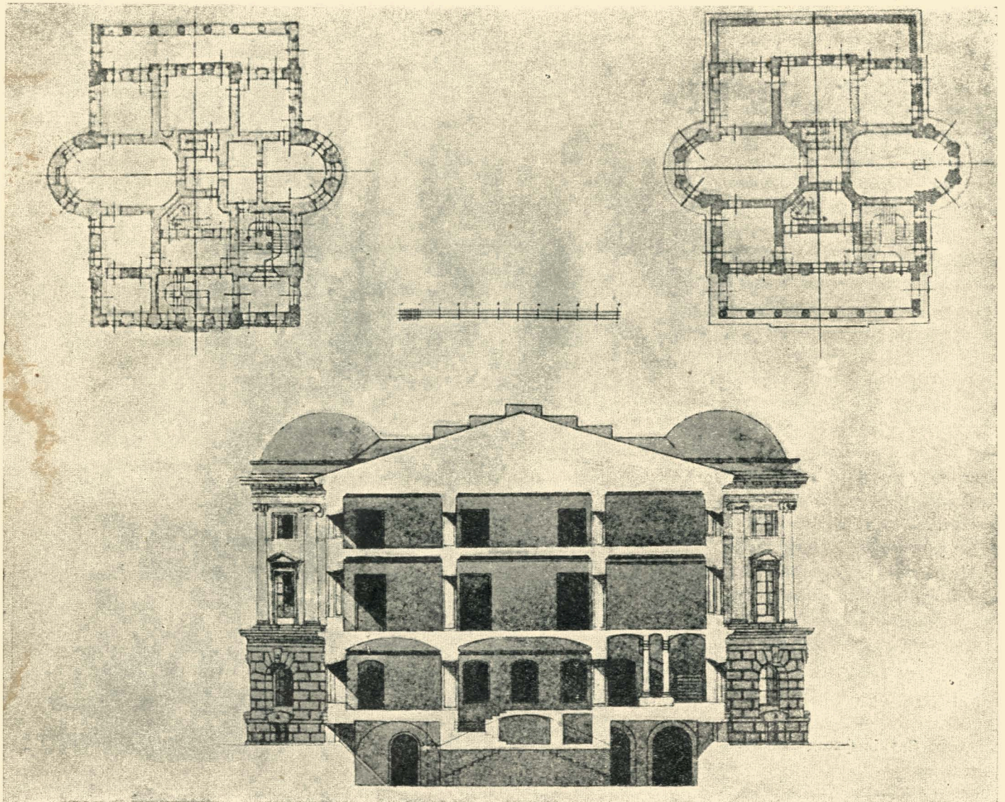
Проект реставрації Батуринського палацу — архітектора А. Белогруда. Розріз і плани.
