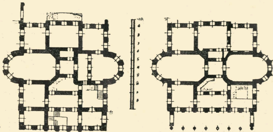
План 1-го і 2-го поверху палацу.
