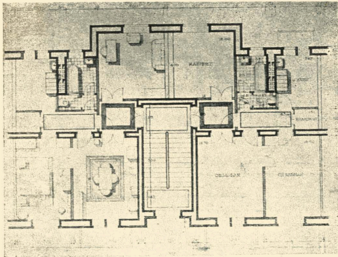
Архіт. Г. Шлаканив і О. Мельнікова (Київ). Проект трикімнатної квартири типу 1938 р. Жила площа — 52 кв. м., k_1 = 0,68 , k_2 = 7,5 .
