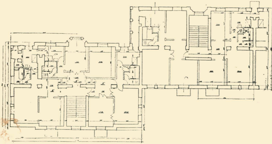
Архіт. І. Михайловський і А. Чечик (Київ). Жилий будинок регенератно-гумового заводу в Києві. Проект дво- і трикімнатних квартир. Жила площа 2-кімн. квартири — 37,69 м 2 , \kappa_1 = 0,61 ; жила площа 3-кімн. квартири — 52,98 м 2 , \kappa_1 = 0,70 , \kappa_2 = 7,4 .
