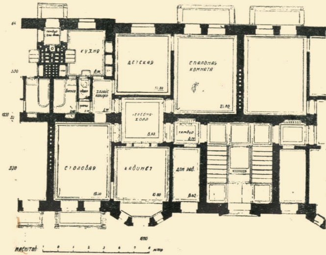
Архіт. Є. Яхненко. Проект 4,5-кімнатної квартири. Жила площа 78,55 м 2 , k_1 = 0,74 , k_2 = 7,5 .
