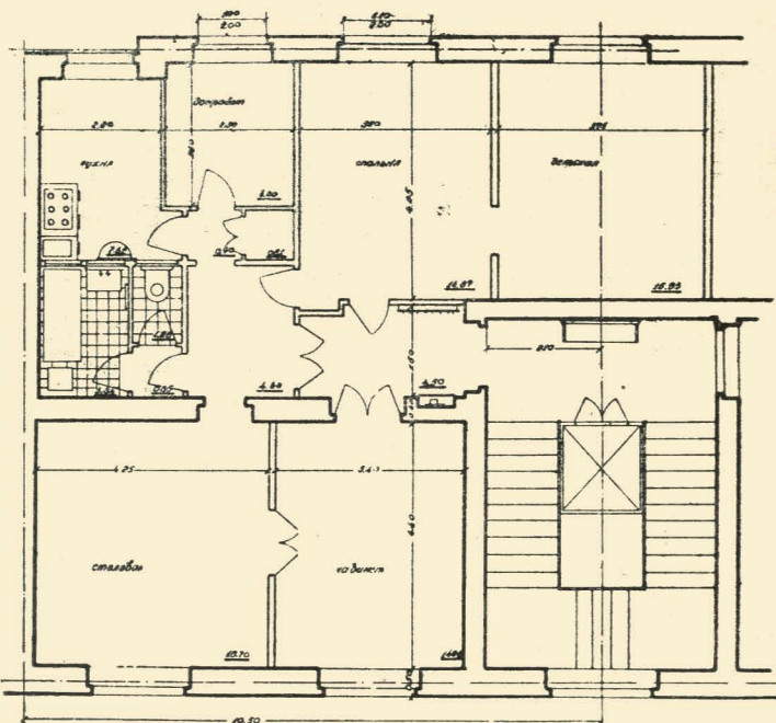
Архіт. Л. Киселевич і І. Хоменко (під керівн. архіт. М. Холостенка—Київ). Проект 3,5 і 4,5 кімнатної квартири. Жила площа 4,5-кімн. квартири—68 м 2 , k_1 = 0,74 . Жила площа 3,5-кімн. квартири 55 м 2 , k_1 = 0,70 .
