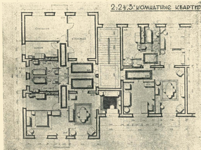
Архіт. Ручко. Проект 2, 2,5 і 3-кімнатних квартир. Жила площа 2-кім. квартири — 36,8 м 2 , k_1 = 0,60 ; жила площа 2,5-кімн. квартири — 45,95 м 2 , k_1 = 0,64 ; жила площа 3-кім. квартири — 55,75 м 2 , k_1 = 0,68 ; об'ємний коефіцієнт k_2 = 7,6 .
