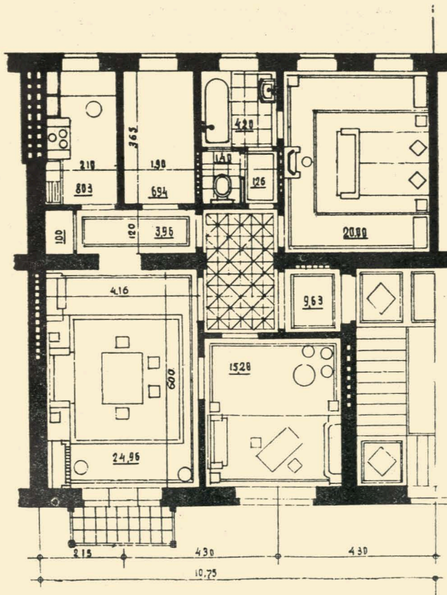
Архіт. Стеценко (Київ). Проект 3,5-кімнатної квартири. Жила площа — 67 кв. м., \kappa_1 = 0,69 .
