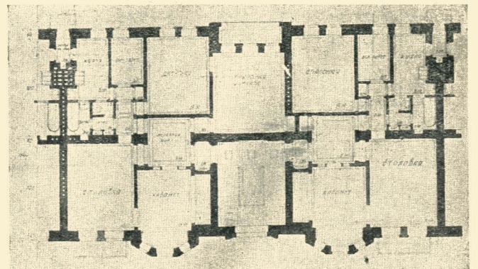
Архит. Є. Яхненко (Київ). Жилий будинок київської міськради на 100 квартир по вул. Кравченка № 6—8 і Глибочицькій № 5—7. Квартири в 3 1/2 кімнати. Жила площа — 61 м 2 , k_1 = 0,70 , k_2 = 7,6 .
