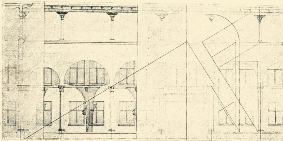
Побудова основних пропорцій внутрішніх фасадів спортивного павільйону.
