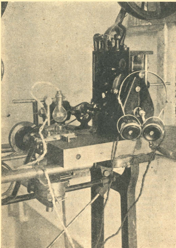
Проекційний звуковий апарат.
