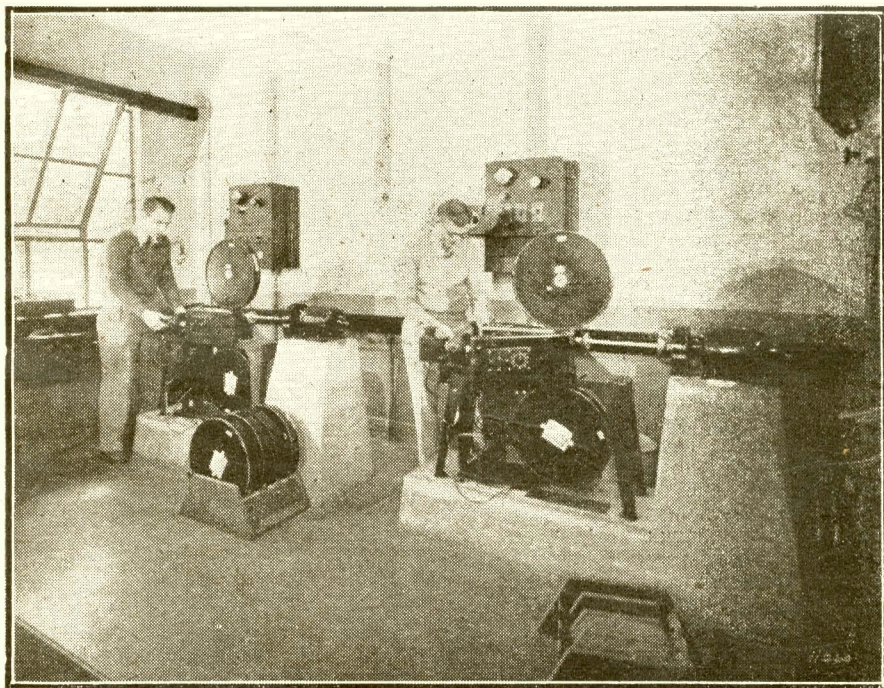
Фотографування звуку. Ці машини реєструють людську мову та інші звуки, що попадають на мікрофон, перетворюючи їх на світляні промені. Система звукового кіна «Метро-Гольдвіна» — найпоширеніша в Америці.
