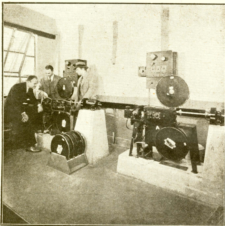
Веслей Мілер, інженер звукового кіна, пояснює систему записів звуку в студіїа „Метро-Гольдвін-Майер“ Сему Вуду—директорові, та Джону Арнольд—операторові. Цей апарат остільки чутливий, що, коли odkривають двері й впускають трошки світла в кімнату, то це вже можна почути, бо апарат реєструє звук через світляний промінь.
