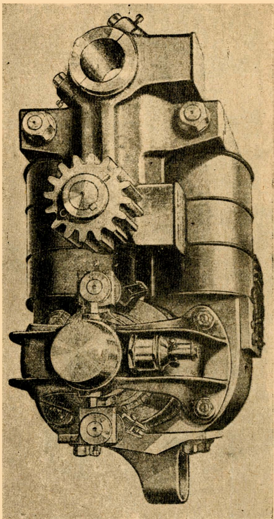
Электромотор «Спрара» (вид сбоку).
