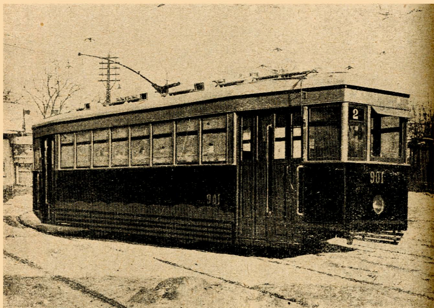
Опытный одноконтроллерный вагон—общий вид.
