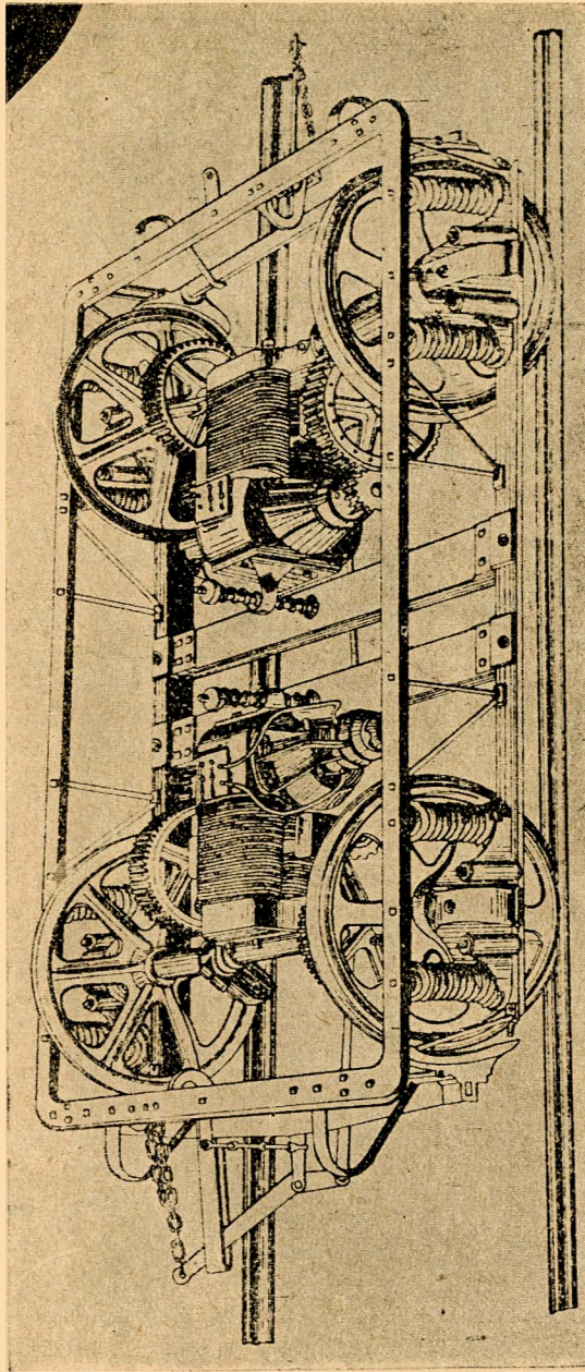
Тележка вагона "Спрага".
