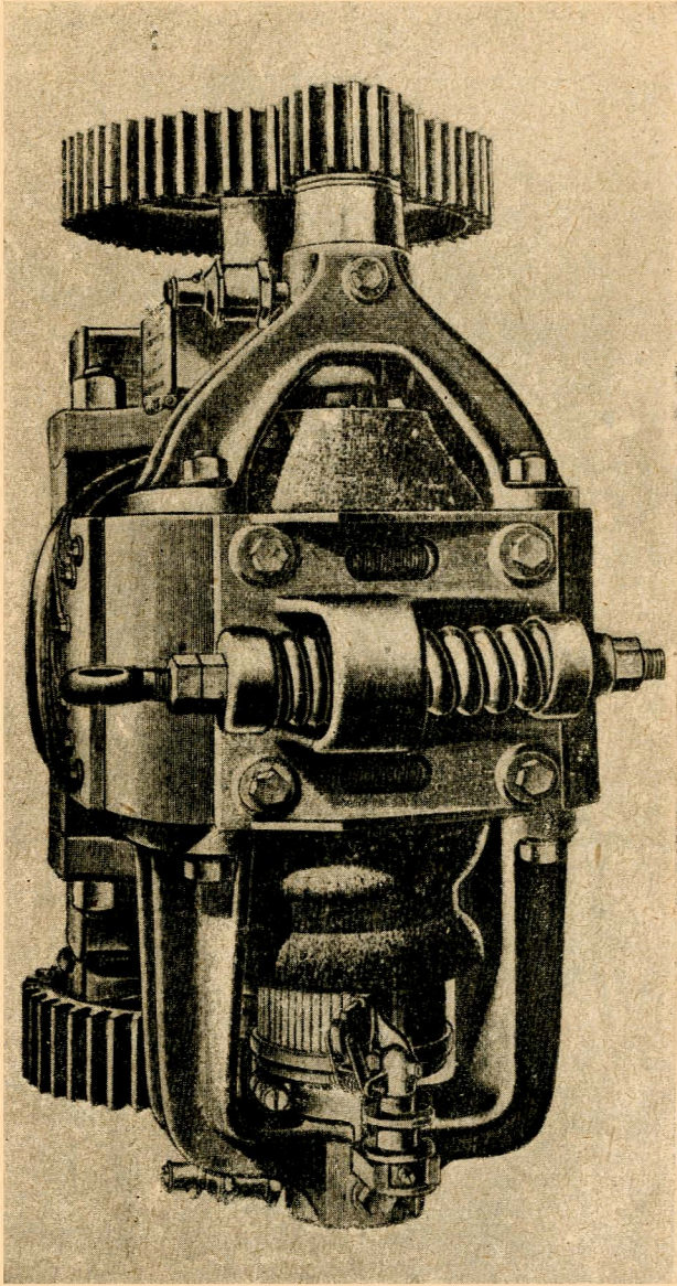
Электромотор „Спрага“ (вид сзади).
