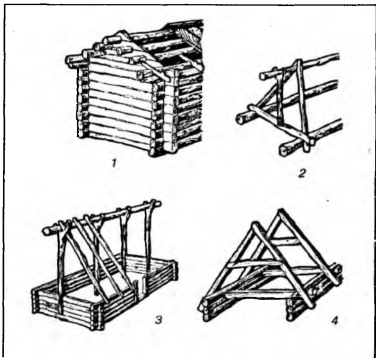
Основні конструкції перекриття у житлово-господарських будівлях: 1 — зрубні дахи; 2 — дахи «на півсохах»; 3 — дахи «на сохах»; 4 — дахи на кроквах
