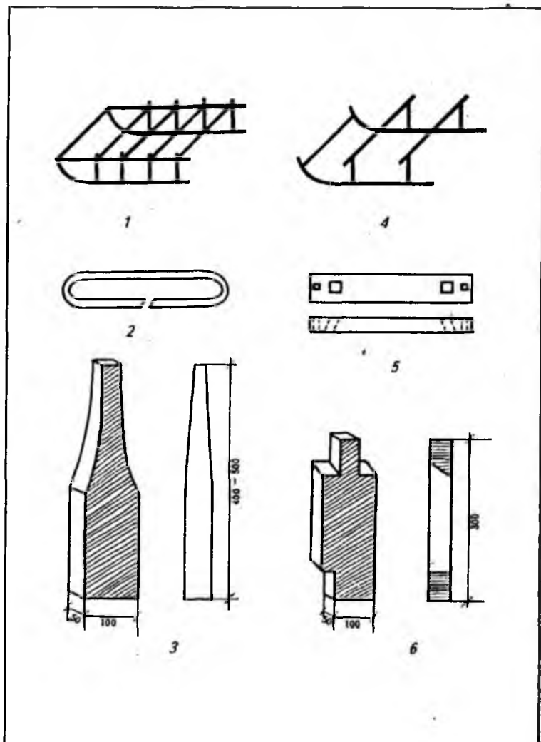
Схеми основної конструкції господарських робочих саней. Східноєвропейські (I): 1 — загальний вигляд; 2 — гнучий «в'яз», що з'єднує полози; 3 — «копило»; західноєвропейські (II): 4 — загальний вигляд; 5 — брусок, що з'єднує полози («насад», «оплін»); 6 — «копило»
