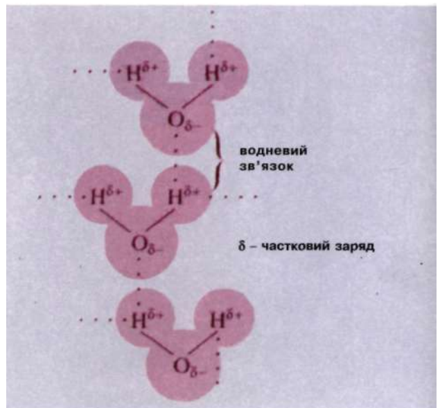
Рис. 1.21 Будова молекули води.
