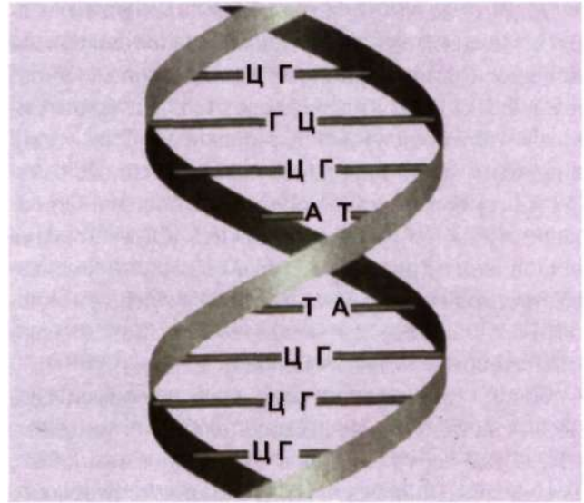
Рис. 1.48 Структура ДНК (фрагмент).
