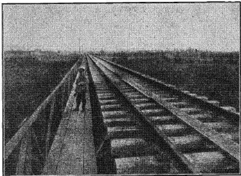
Як Німці будують залізничні шляхи на занятих болотистих землях в російській Польщі.
