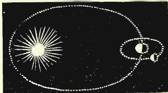
Обіг землі довкола сонця по дорозі, по якій крутив ся колєсь відірваний від сонця обруч. Довкола землі знова обігає по тій самій причині місяць.
