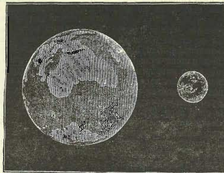
Земля і місяць та їх величина.
