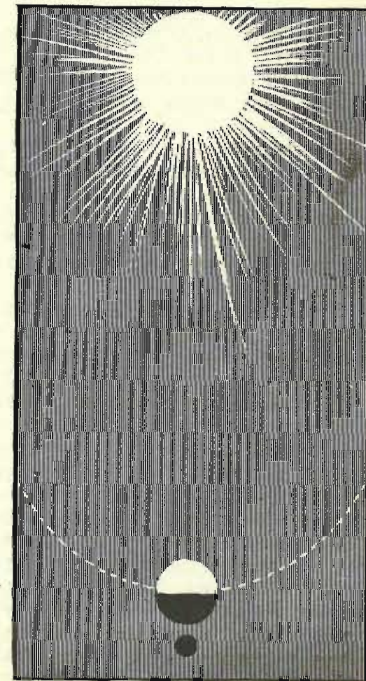
Ніч і день на землі.
