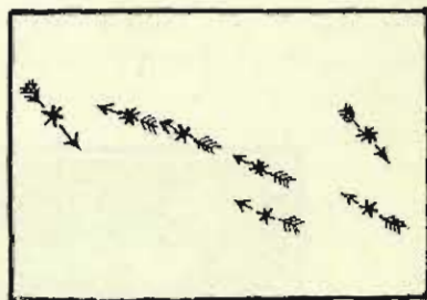
Рух зьвізд в Великім Возі.
