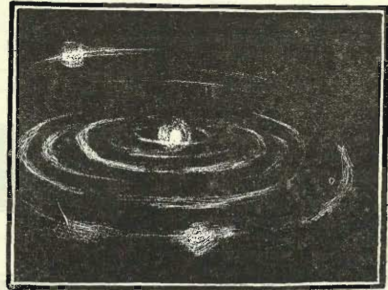
Творене ся планет і сонця.
