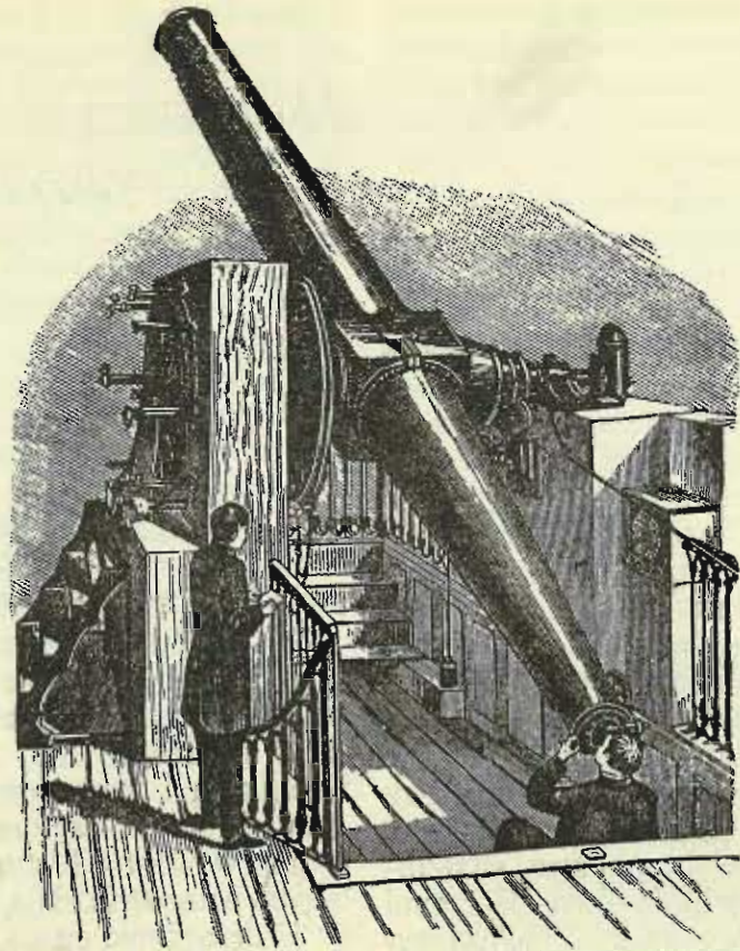
Дальновид, крізь які глядять астрономи на зьвізди.
