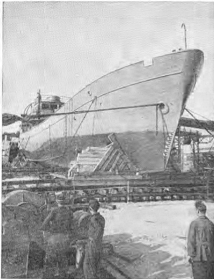
Будівництво морських дизельних траулерів на заводі «Ленінська кузня».
