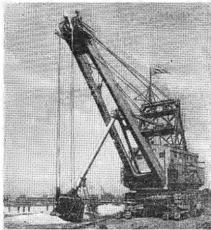
Крокуючий екскаватор Ново-Краматорського заводу ім. Сталіна.
