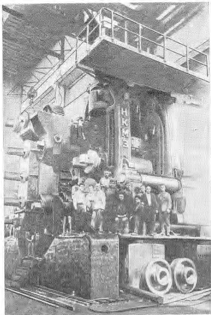
Перший слябінг, виготовлений Ново-Краматорським машинобудівним заводом.
