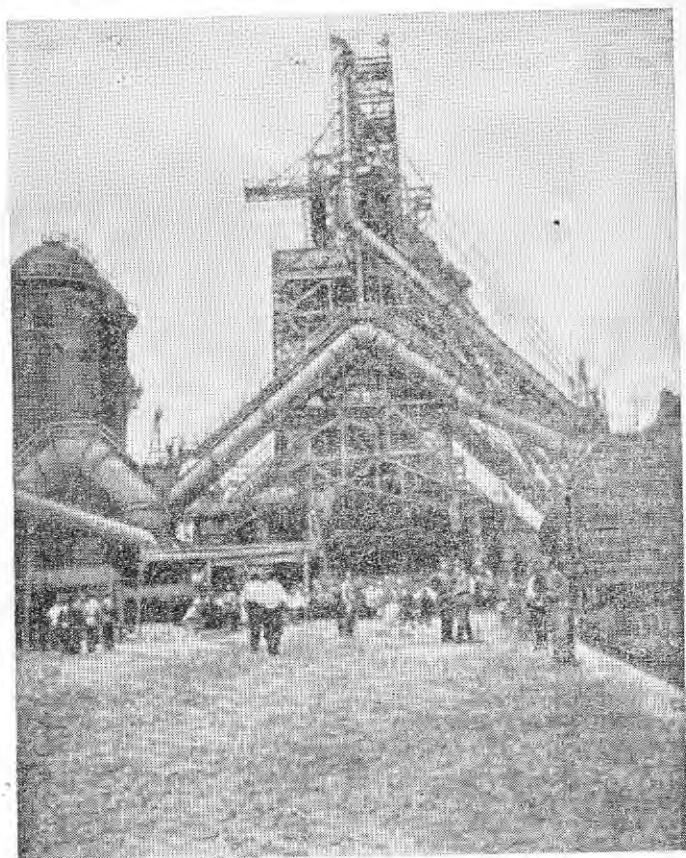
Новозбудована домна № 2-біс на Краматорському машинобудівному заводі (1927 р.).
