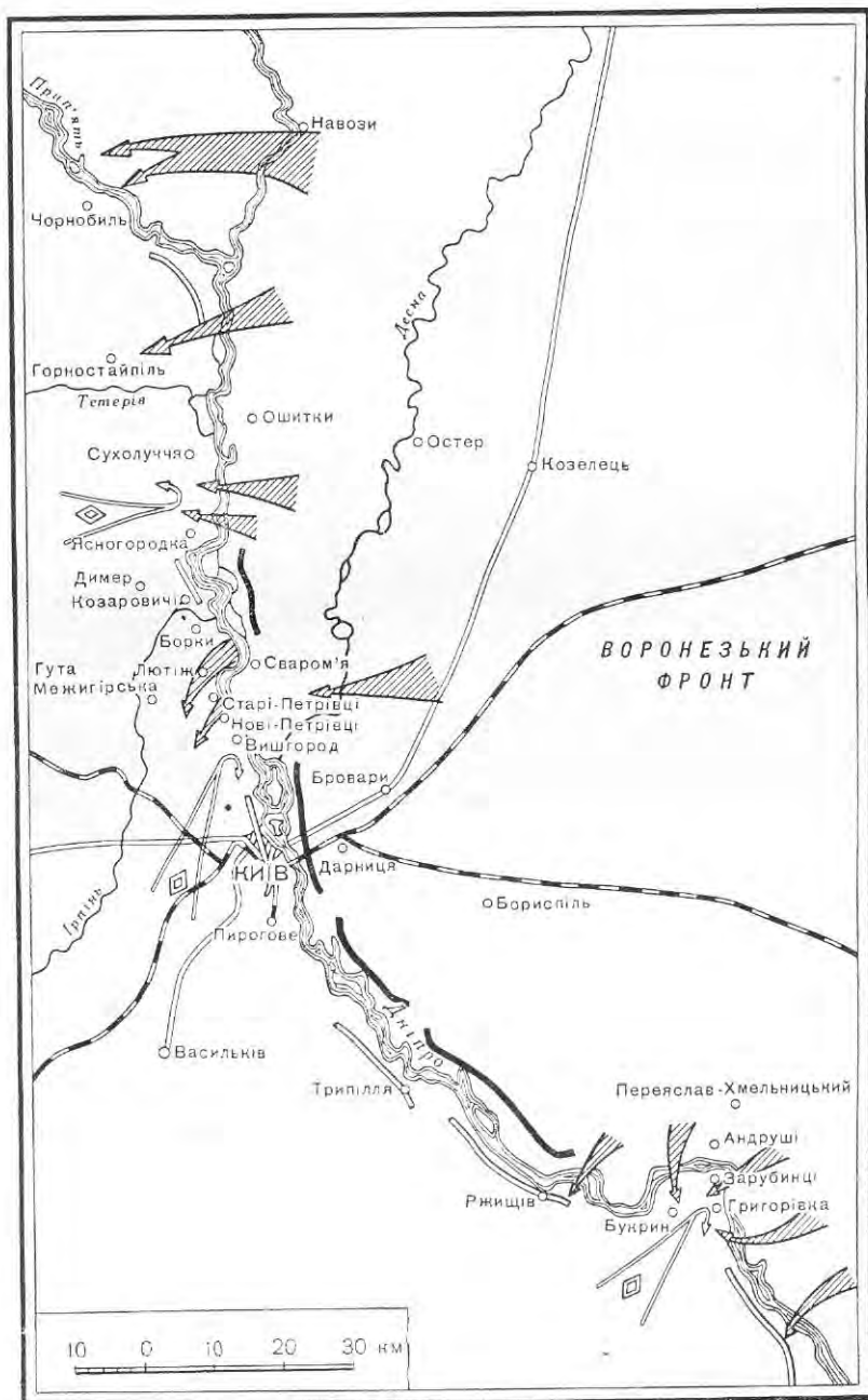
Схема форсування Дніпра військами Воронежського фронту.
