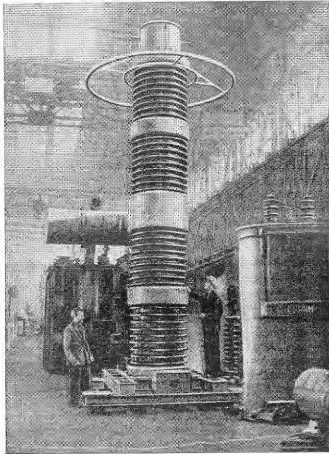
Виготовлення трансформаторів на Запорізькому трансформаторному заводі для високовольтної лінії електропередачі Куйбишев — Москва.
