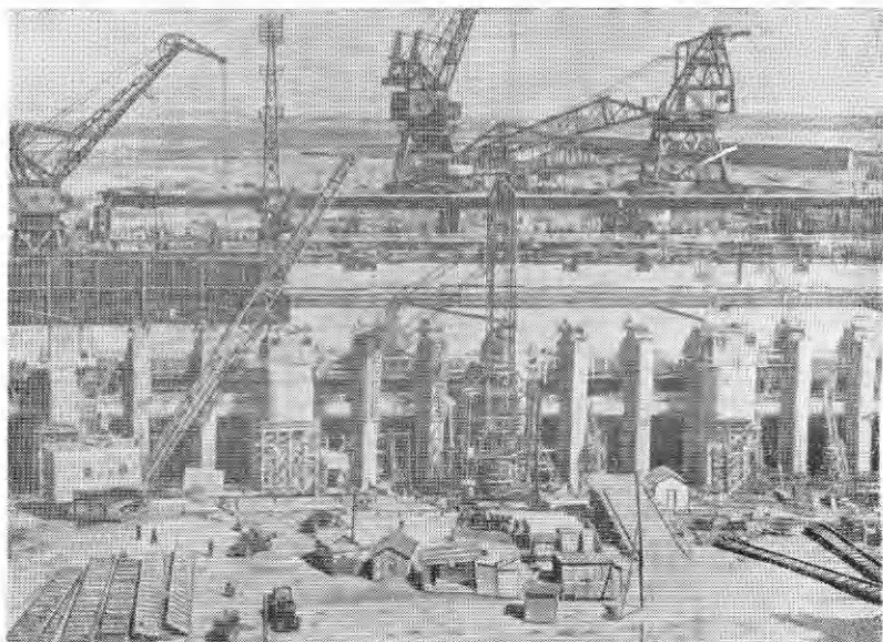
Будівництво Каховської гідроелектростанції (1953 р.).
