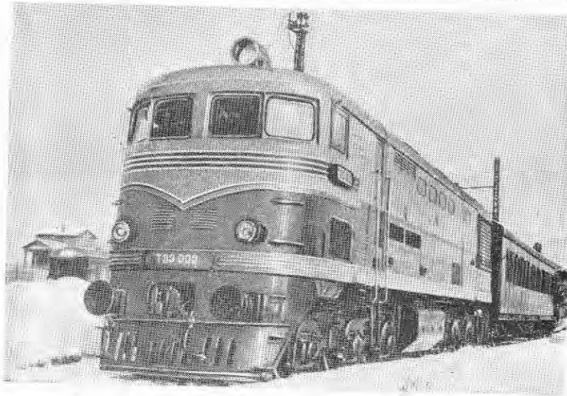
Тепловоз ТЭ-3 Харківського паровозобудівного заводу.
