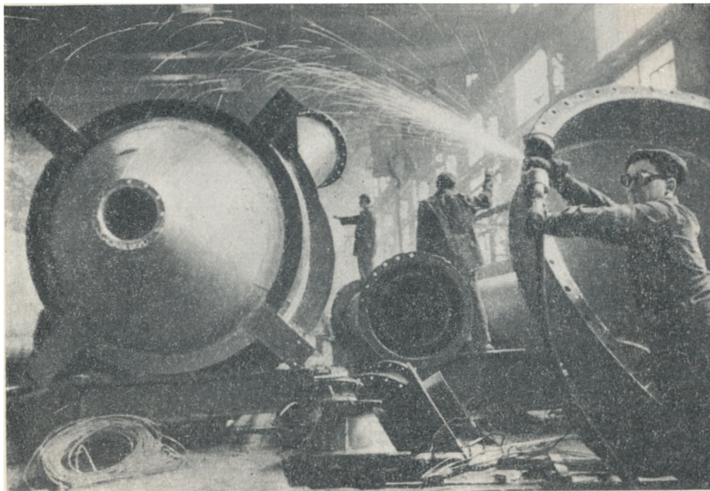
На заводі металокопструкцій ім. І. В. Бабушкіна. Складальний цех.
