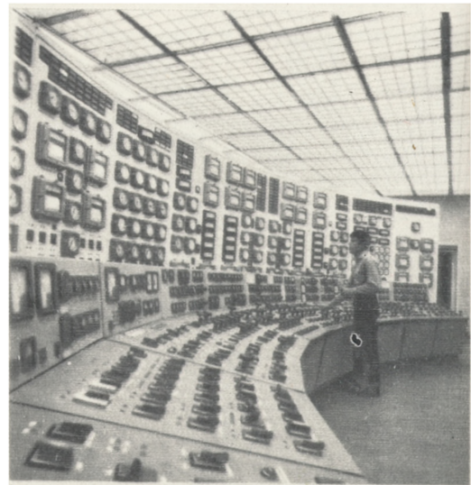
Придніпровська ДРЕС. Блочний щит управління.
