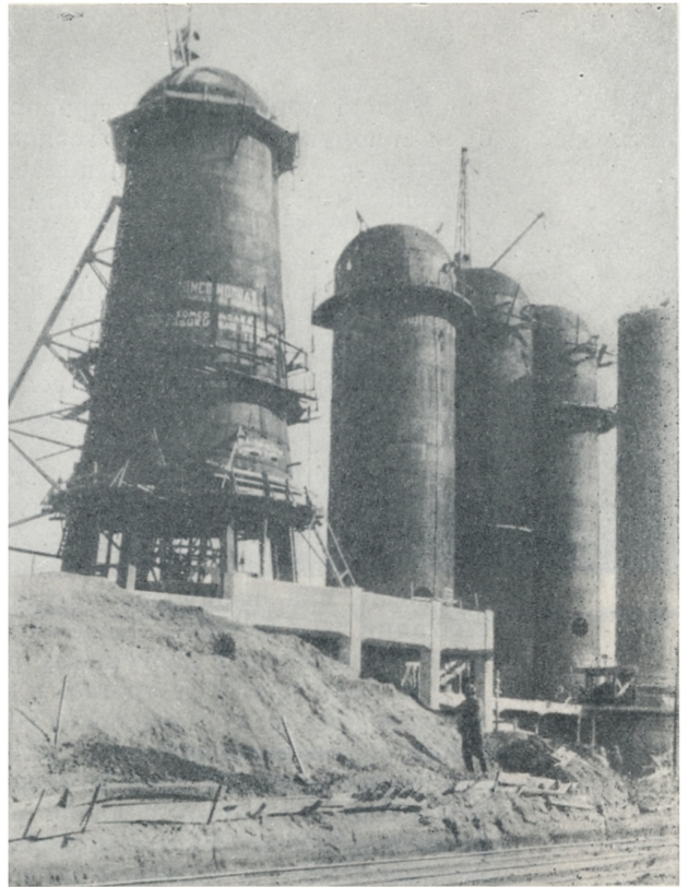
Домна «Комсомолка», збудована в 1931—1934 рр. Кривий Ріг.
