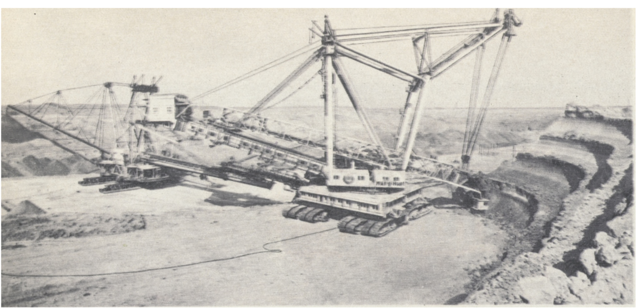
Роторний екскаватор. Кар'єр Грушівського рудо-управління тресту «Нікопольмарганець».
