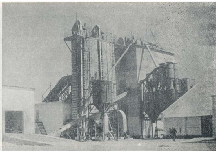
Потокова система Щорського кукурудзокалібрувального заводу. 1966 р.
