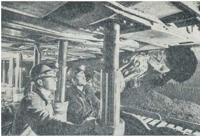
Автоматичний вугледобувний комплекс КМ87-АЕ в одній з лав шахти № 3 «Добропілля». 1968 р.
