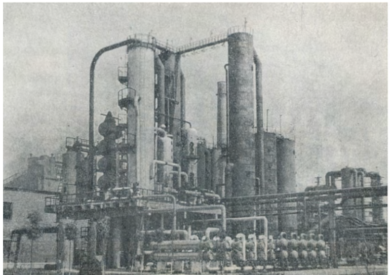
Бензолне відділення Авдіївського коксохімічного заводу. 1965 р.
