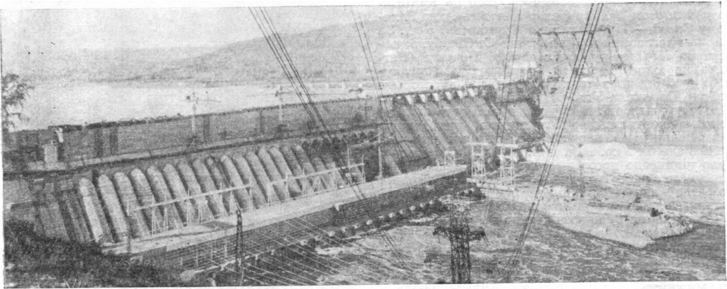
Красноярська ГЕС. 1970.
