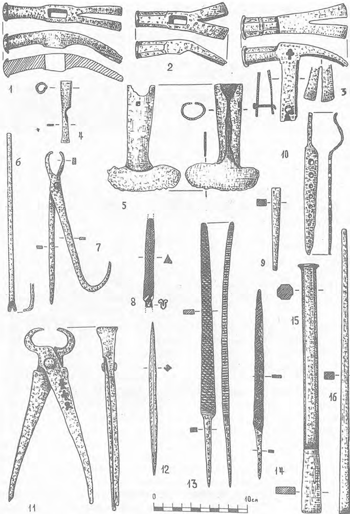
Р и с. 46. Залізни інструменти з козацької перепази.
