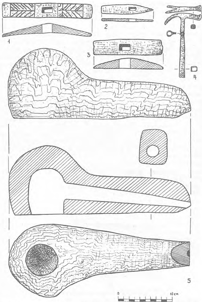
Рис. 48. Залізні молотки (1—4) і дерев'яна частина апарату до «куріння» горілки (5) з козацької переправи.
