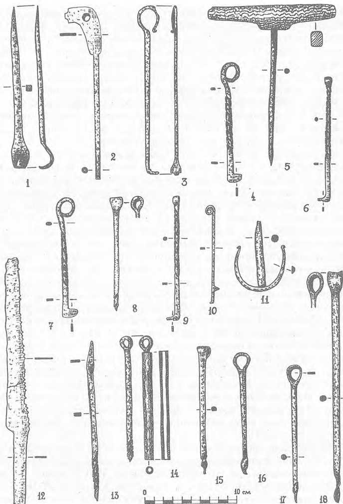
Р и с. 47. деревообробні інструменти з переправи.
