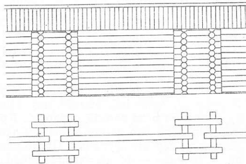
Схема конструкції стіни на зрубів-«столпах». Фасад і план.
