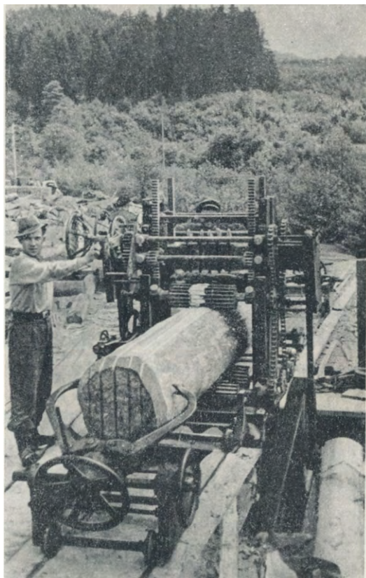
Пилорама керецьківського колгоспу «Пам'ять Ілліча». 1967 р.
