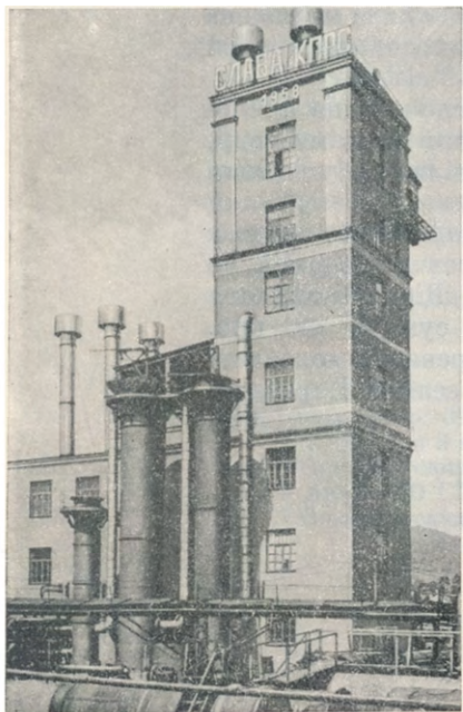
Реторта Перечинського лісохімкомбінату. 1967 р.
