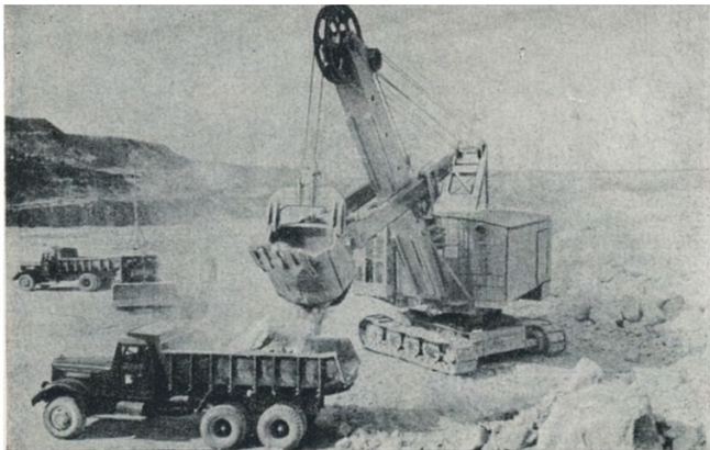
Видобуток і навантаження флюсового вапняку. Балаклавське рудоуправління. 1954 р.
