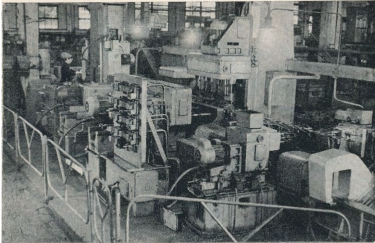
Автоматична лінія для обробки корпусів масляних насосів Кіровоградського заводу тракторних гідроагрегатів. 1971 р.
