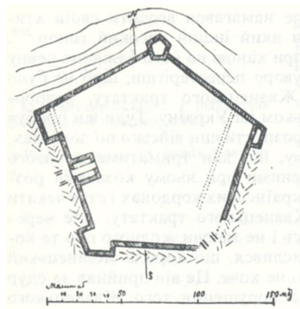
Замок у Жванці.— План (43).
