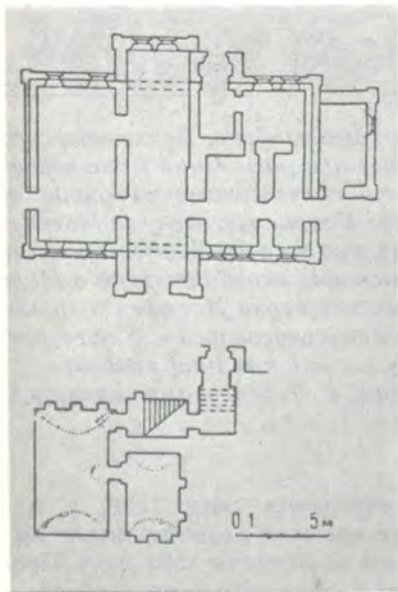
Будинок В. Кочубея в Батурині. XVII ст. План наземного поверху (62).
