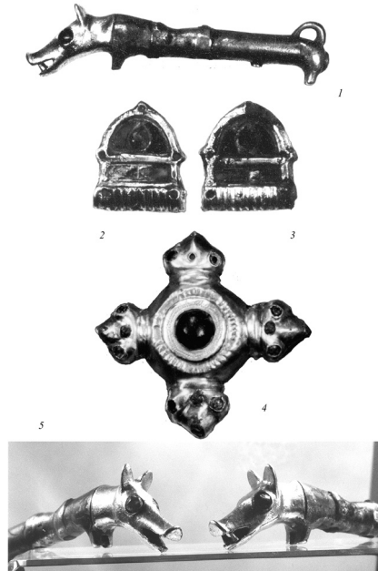
Рис. 3. Уздечный набор 1. 1, 5 — псалии, 2–4 — фиксаторы ремней оголовья
