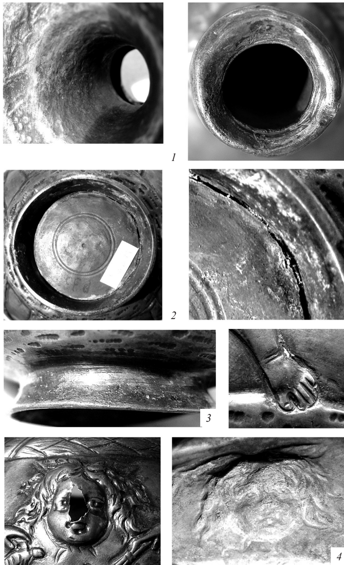
Рис. 2. Серебряный сосуд, гробница Рискупорида. Керчь, III в. н. э.: 1 — следы выколотки и правки на токарном станке на крышке; 2 — припаянное дно, завальцованное на токарном станке; 3 — следы подработки на токарном станке на поддоне; 4 — чеканный орнамент
