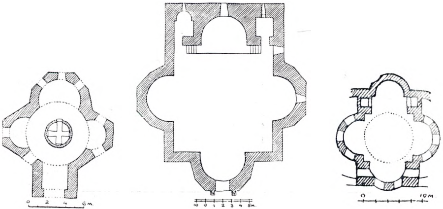
9. Схема внутрішнього просторового об'єму середньої частини Сугківської твердині. — 10. План баптистерія в Херсонесі 600 р. — 11. План церкви в Mastara VII ст. — 12. План „Червоної церкви“ в Пловдиві IX ст.
