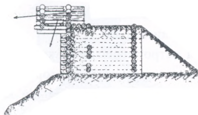
Дерево-земляне укріплення з бойовою галереєю за В. Яковлевим. Стрілками показано напрями обстрілу
