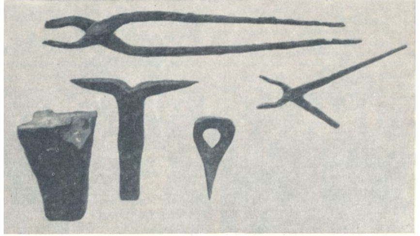
257. Ковальські інструменти. Ковадла, кліщі, зубило. Родень.
