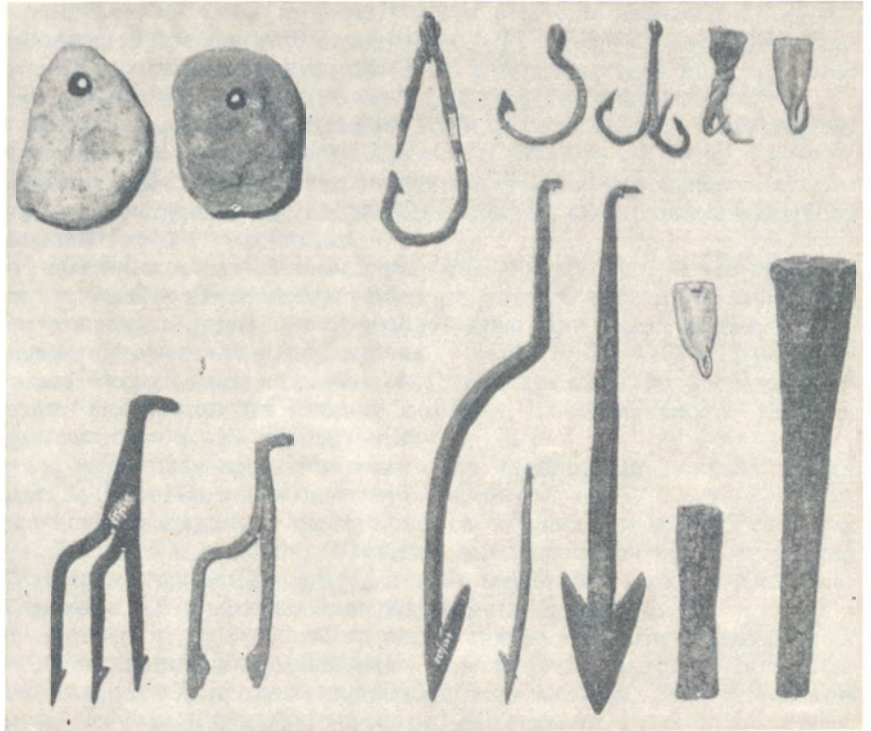
162. Рибальське знаряддя. Грузила, гачки, блешні, ості, гарпун, плішні. Родень.
