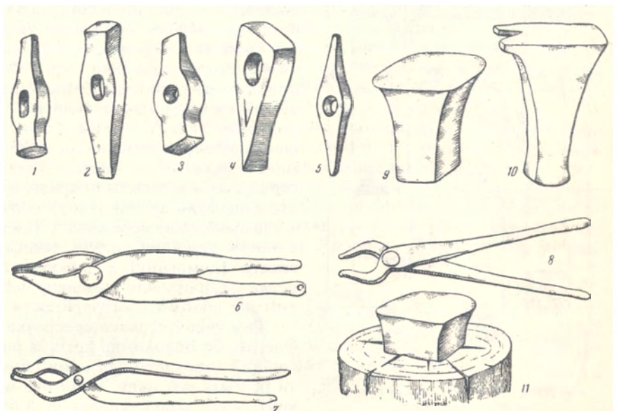
258. Ковальські інструменти.
