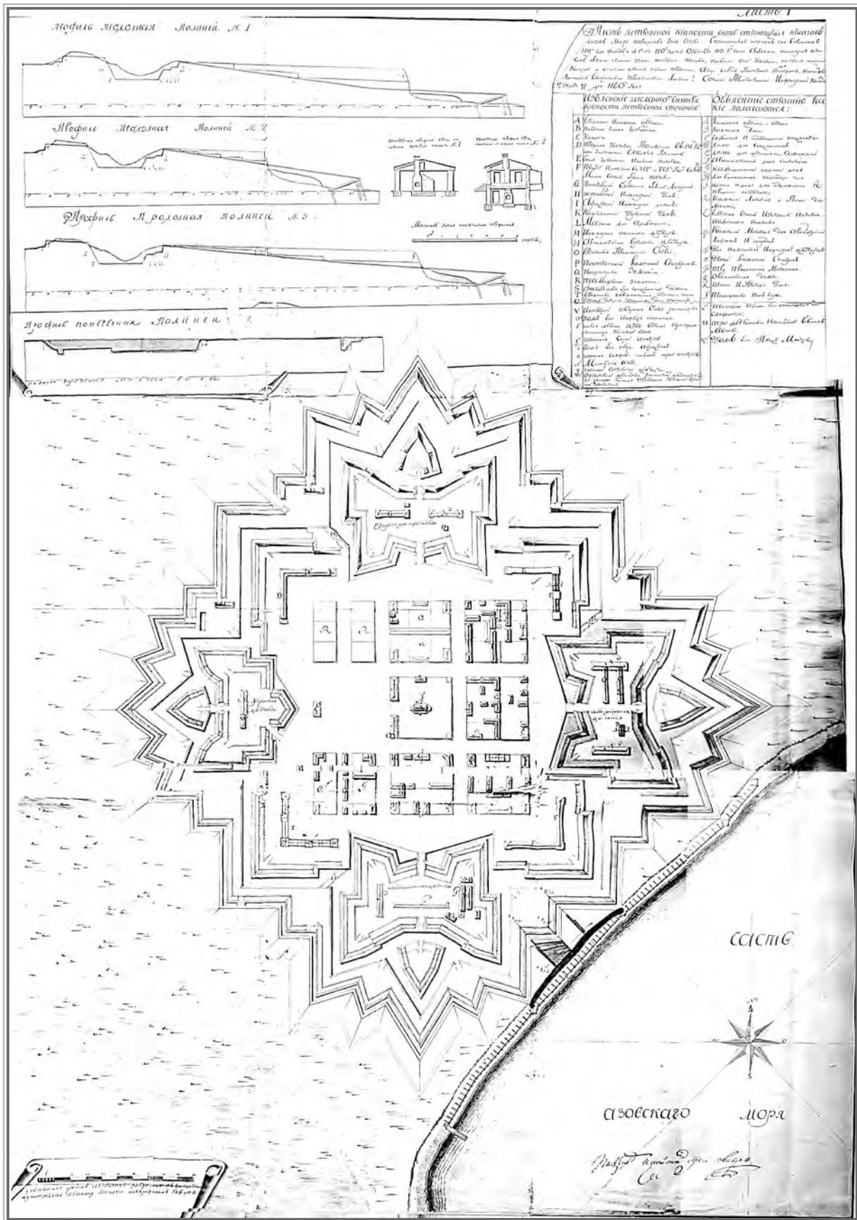
Крепость Петровская. 1780 г. ГААРК, ф. 535, оп. 1, д. 3151
