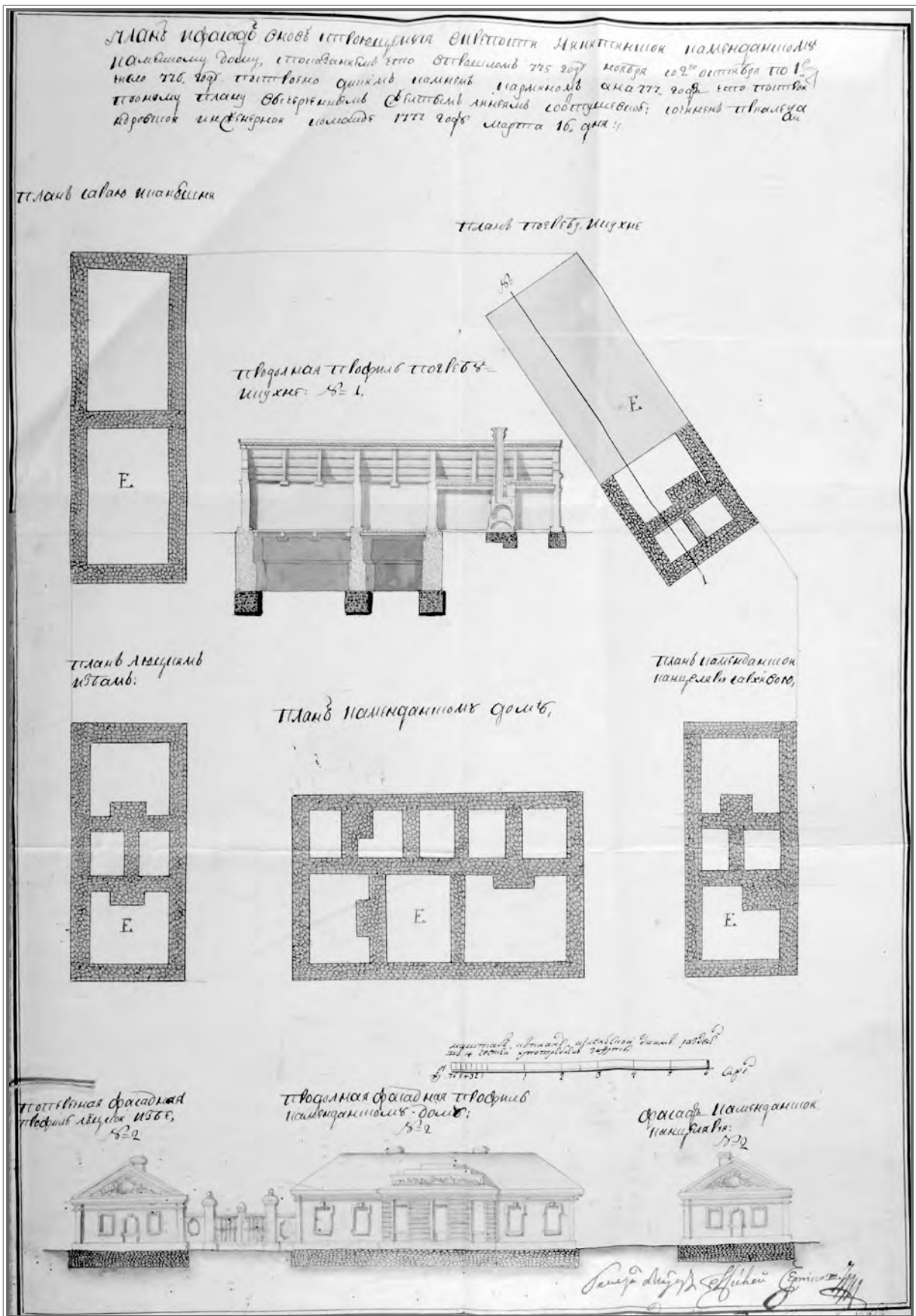
План и фасад командантского дома в крепости Никитинской. 1777 г. ГААРК, ф. 535, оп. 1, д. 3146
