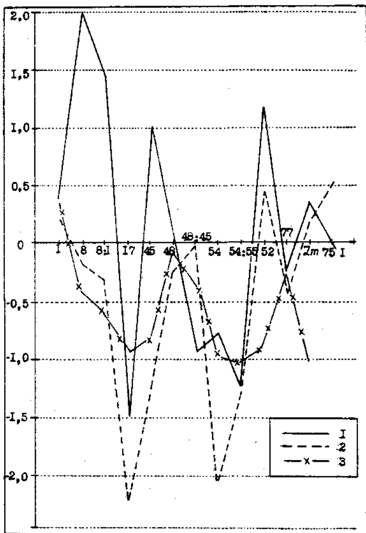
Рис. 37. Сопоставление женских черепов сарматов Правобережной Украины с синхронными позднесарматскими сериями: 1 – бассейн р.Молочной; 2 – Усть-Каменский могильник; 3 – Золотобалковский могильник
