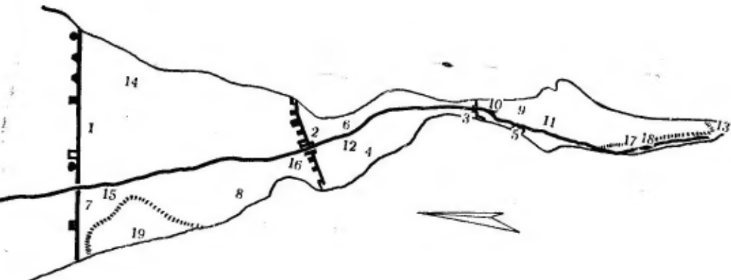
Рис. 2. План крепости на мысе Калиакра с раскопанными археологическими объектами: 1—первая укрепительная линия; 2—вторая укрепительная линия; 3—третья укрепительная линия; 9—10—средневековый внутренний город. Останки фрако-эллинистического укрепительного поселения Тиризис и римско-византийской цитадели
