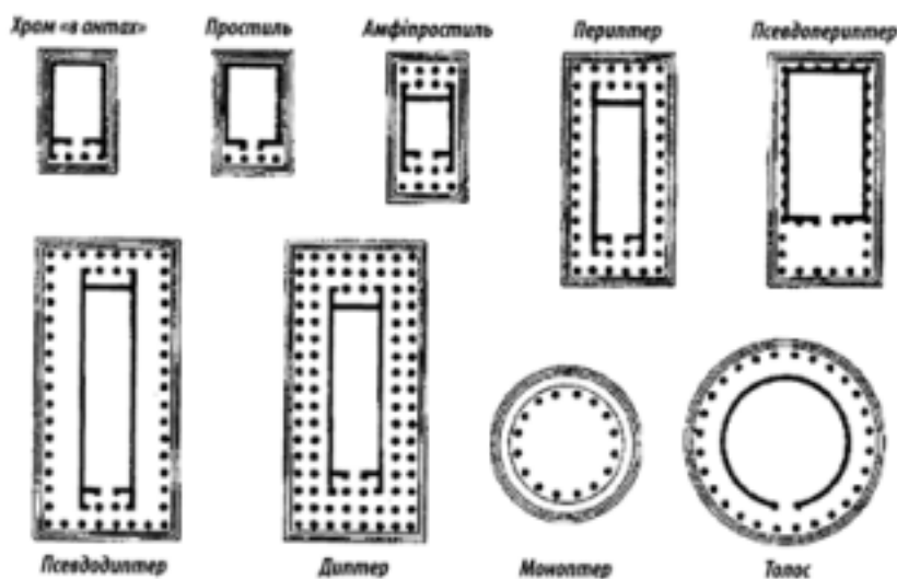
Типи грецьких храмів
