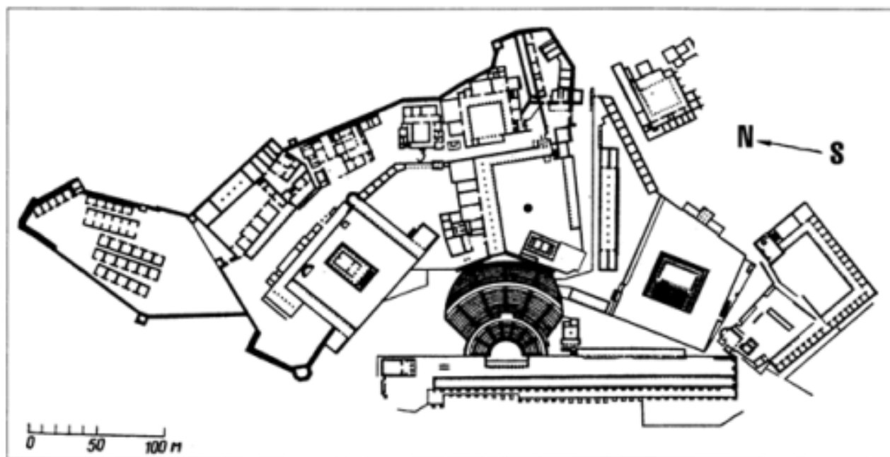
Пергам. План акрополя
