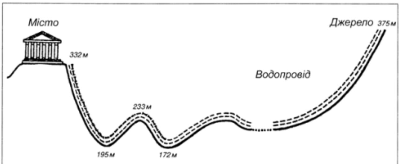
Схема пергамського водопроводу
