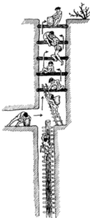
Шахта з видобутку руди
