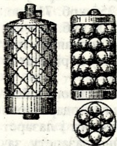
Снаряд-шрапнель гладкоствольної артилерії.
