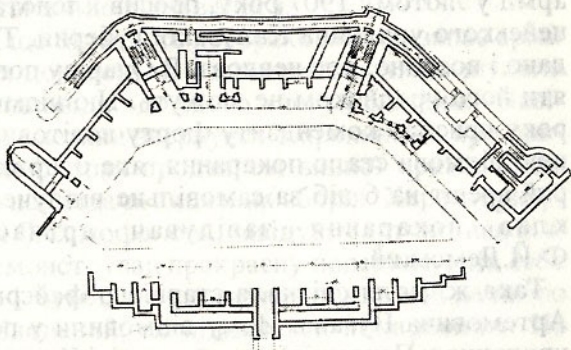
План розміщення безпечних казематів. II-й поверх.
