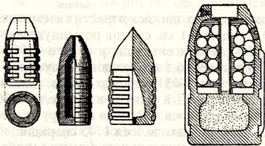
Снаряди до гармат зразка 1867 року.
