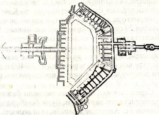
План розміщення безпечних казематів форту. 1-й поверх.
