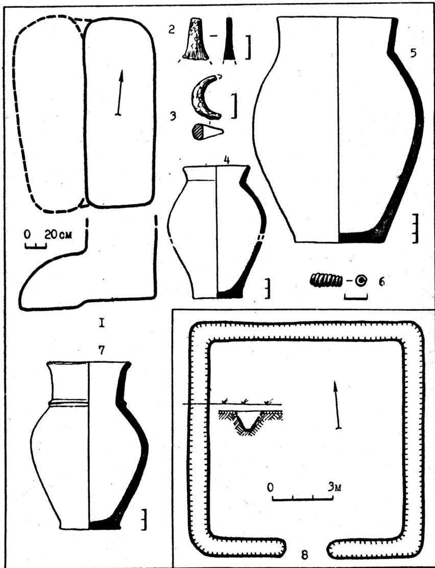
Рис.8. Васильевский могильник. Курган 26: I-7 - погребение 2 и вещи из него. Ров I: 8 - план (2,3 - железо; 4,5,7 - керамика; 6 - бронза, железо).
