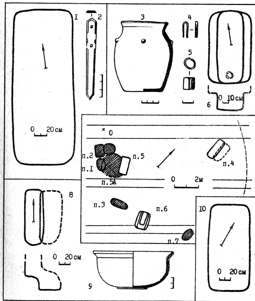
Рис.3. Васильевский могильник. Курган I: 1,2 - погребение 2 и оконцовка из него; 3-6 - погребение 3 и вещи из него. Курган 6: 7 - план кургана; 8,9 - погребение 4 и миска из него; 10 - погребение 5 (2 - бронза, железо; 3,9 - керамика; 4,5 - бронза).
