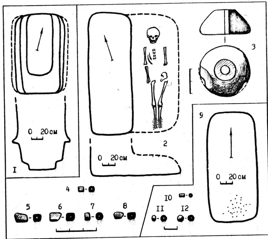
Рис.4. Васильевский могильник. Курган 6: I - погребение 6. Курган II: 2-8 - погребение I и вещи из него; 9-12 - погребение 2 и бусы из него (3 - глина; 4-8,10-12 - стекло).
