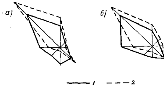
Рис. 5. Орографические розы ветров в 13 час. (1) и 1 час (2). а — Каменец-Подольский, б — Могилев-Подольский.
