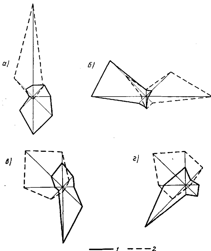
Рис. 6. Розы ветров при бризах в 13 час. (1) и в 1 час (2). Июль. а — Карадаг, б — Севастополь, в — Одесса, обсерватория, г — Скадовск.
