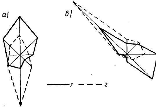
Рис. 4. Розы горно-долинных ветров в 13 час. (1) и в 1 час (2). а — Селятин, б — Ай-Петри.
