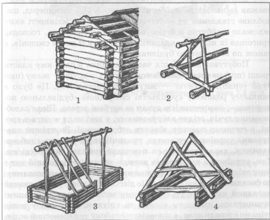
Основні конструкції перекриття у житлово-господарських будівлях:
