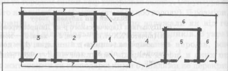
Зімкнутий тип забудови двору («хижка під одним побоєм»)
