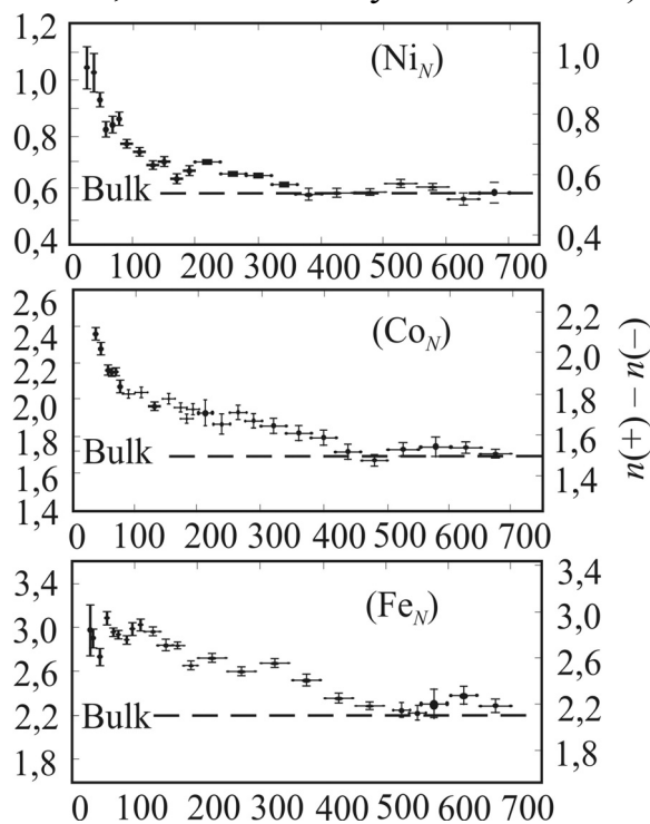
Рис. 4.6. Магнітний момент, розрахований на один атом для феромагнетиків Ni, Co і Fe залежно від розміру частинок в ангстремах (1 А = 0,1 нм; bulk)
