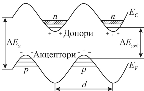
Рис. 4.32. Енергетичні діаграми легованої надгратки: \Delta E_{gef} – ефективна ширина забороненої зони надгратки; d – її період
