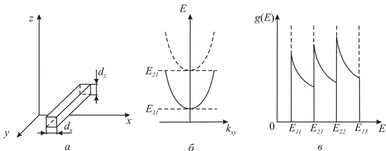
Рис 4.20. Одновимірний (1D) нанооб'єкт – квантовий дріт:
