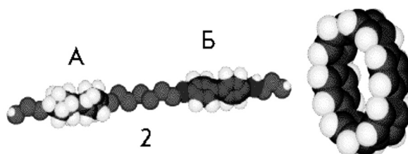
Рис. 4.47. Логічний елемент на основі молекул ротаксану: 1 – циклічний компонент, або «бусина»; 2 – лінійний компонент, або «нитка».
