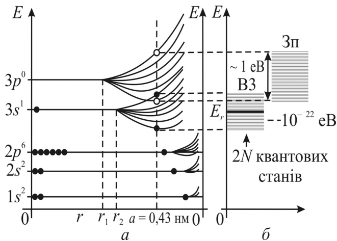
Рис. 3.19. Енергетичні спектри: а – окремого атома натрію; б – системи N атомів залежно від відстані між ними; ЗП – зона провідності; ВЗ – валентна зона
