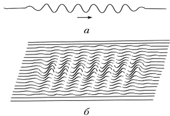
Рис. 3.5. Хвильовий пакет: а – одновимірне подання; б – двовимірне подання
