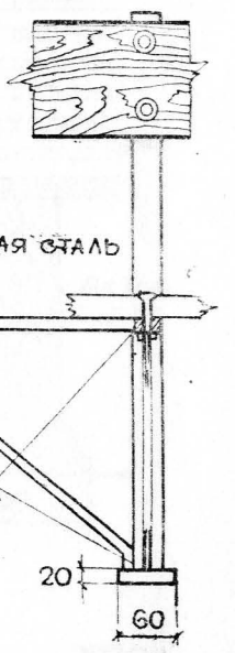
РАЗРЕЗ 2-2
