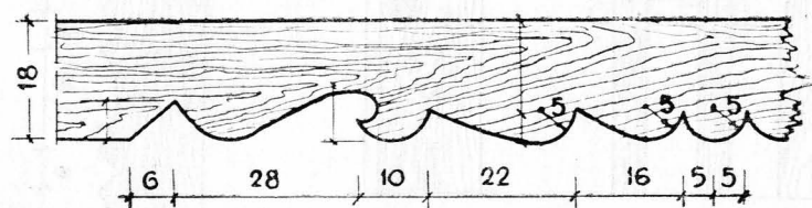
ПОРЕЗКА ДОСОК ЗАБОРА "Е"
