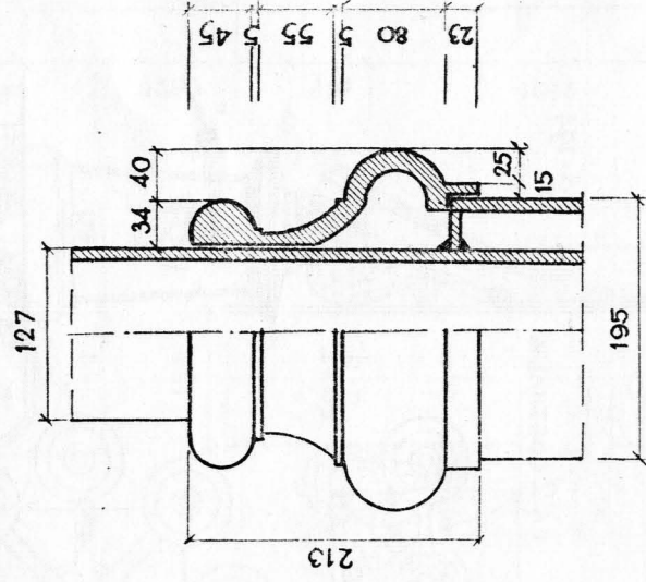
ДЕТАЛЬ "В"
