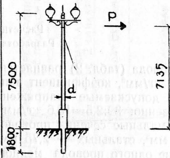
15,16. ОПОРЫ - СТАЛЬНЫЕ ТРУБЫ
