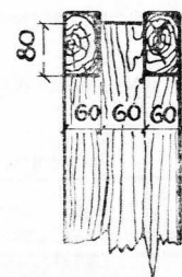
ВИД ПО 1-1
