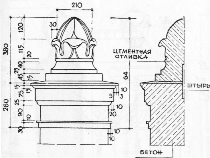
ДЕТАЛЬ „А“
