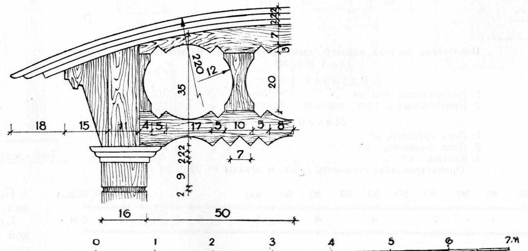
„В“ ПОРТАЛ КАЛИТКИ
