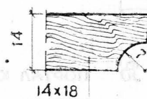
ДЕТАЛЬ ВОРОТ "В"
