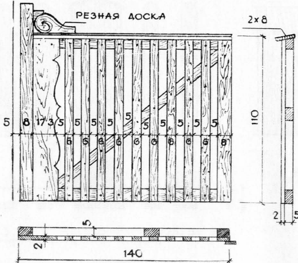
А ВОРОТА
