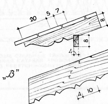
ДЕТАЛЬ "Б"
