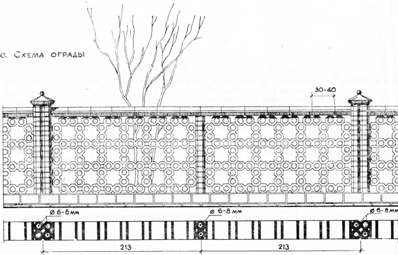
в. СХЕМА ОГРАДЫ
