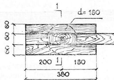
ВИД ПО 1-1
