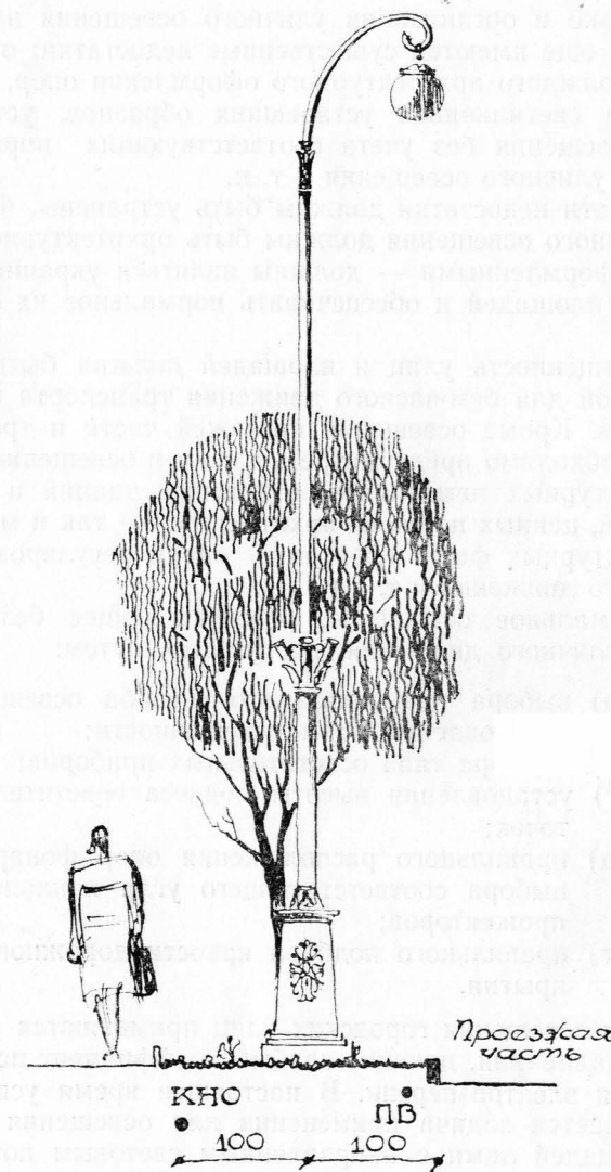
Рис. 3. Установка фонаря в поперечном профиле улицы.
