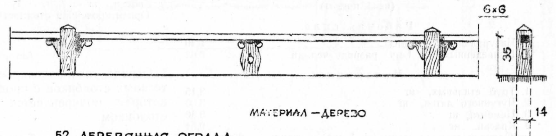
52. ДЕРЕВЯННАЯ ОГРАДА
