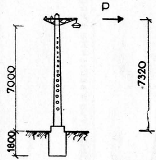
13,14. ОПОРЫ - ДЕРЕВЯННЫЕ СТОЛБЫ
