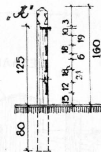
РАЗРЕЗ а-а
