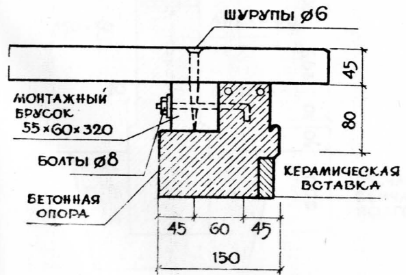
СЕЧЕНИЕ 2-2
