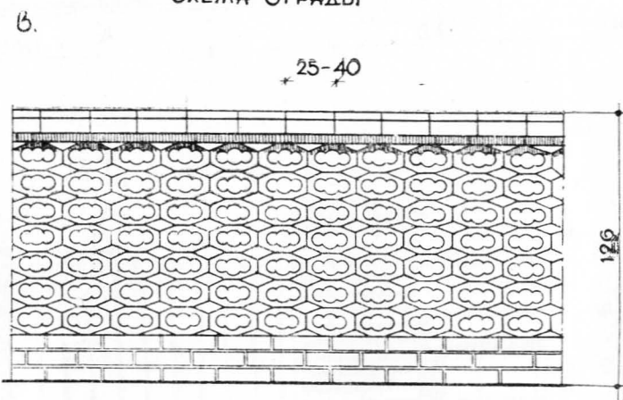
СХЕМА ОГРАДЫ
