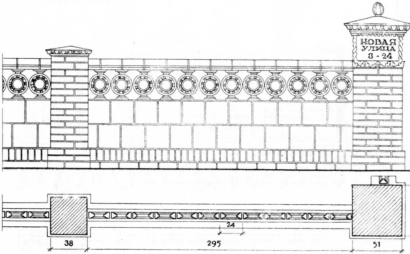
СХЕМА ОГРАДЫ "Д"
