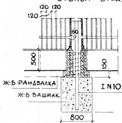
ДЕТАЛЬ "Ж"
