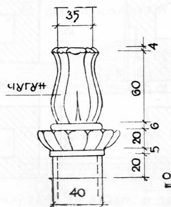
"В" ДЕТАЛЬ ПОРТАЛА
