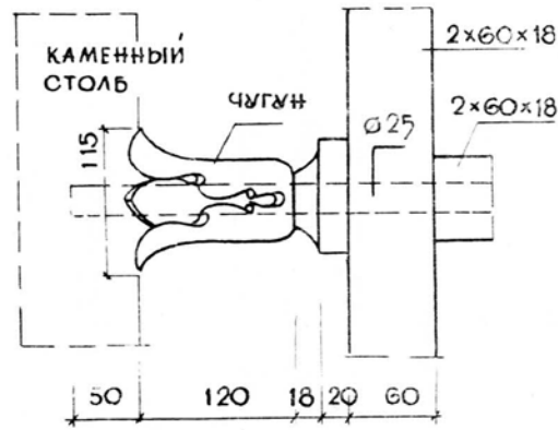
ДЕТАЛЬ „Д“
