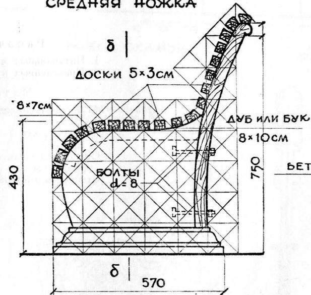
СРЕДНЯЯ НОЖКА
