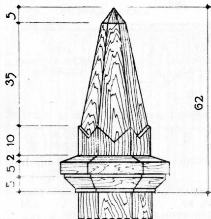
"А" ДЕТАЛЬ ОГРАДЫ
