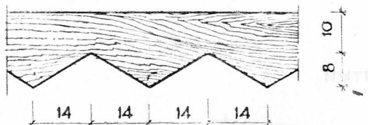
ПОРЕЗКА ДОСКИ ПОД КРЫШЕЙ "Б"
