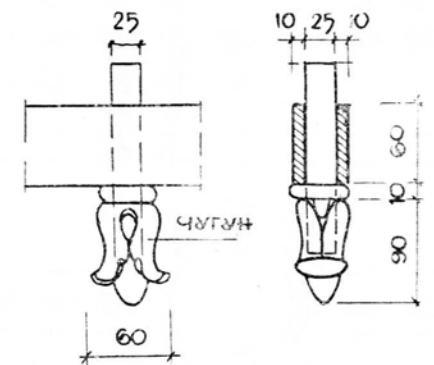
ДЕТАЛЬ „Г“
