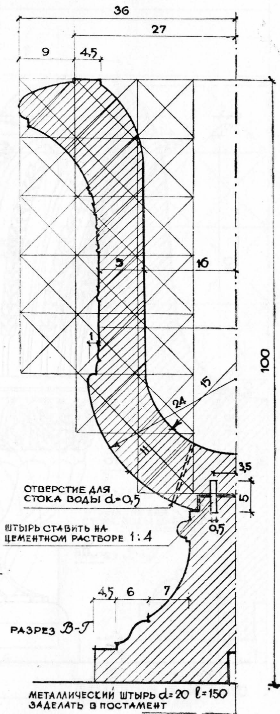
РАЗРЕЗ ПО ВЕРТИКАЛЬНОЙ ОСИ
