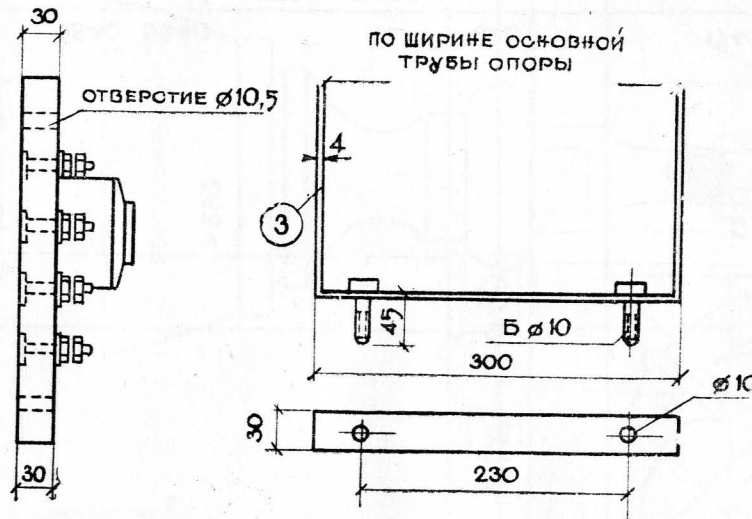
СКОБА ДЛЯ КРЕПЛЕНИЯ ВОРОНКИ
