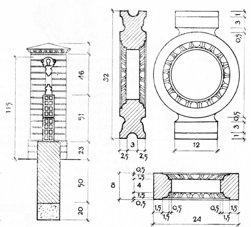
КЕРАМИЧЕСКИЕ ПОРУЧНИ
