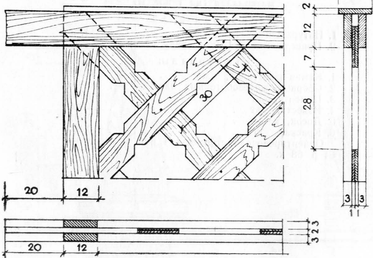
„А“ ДЕТАЛЬ ОГРАДЫ
