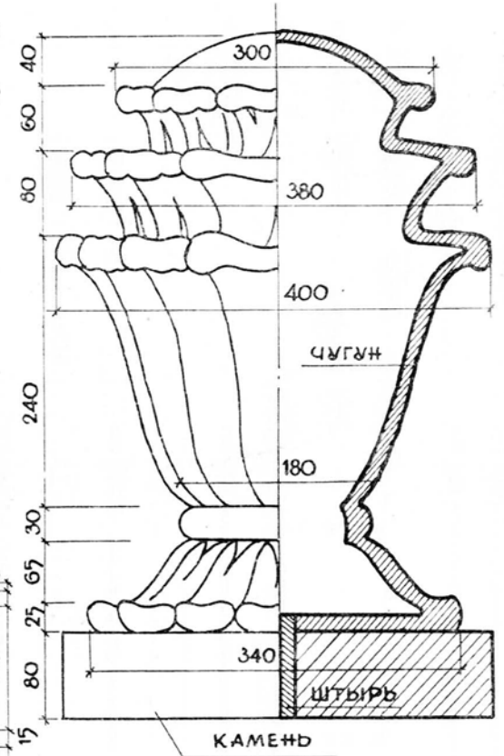
ДЕТАЛЬ „Г“
