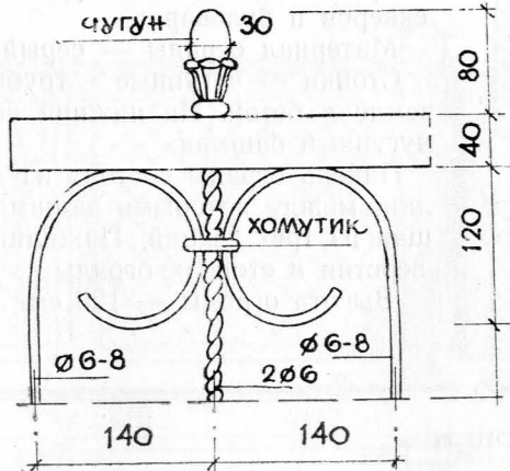
"Б" ДЕТАЛЬ ОГРАДЫ
