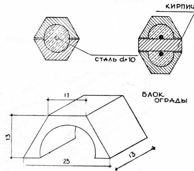
СХЕМЫ СТОЛБОВ
