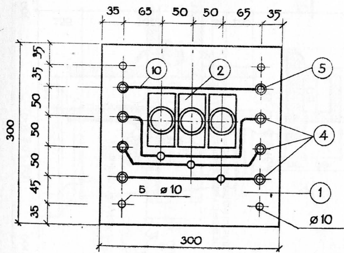
КАБЕЛЬНАЯ ВОРОНКА ДЛЯ КАБЕЛЯ 1 кв. 10-16 кв.мм
