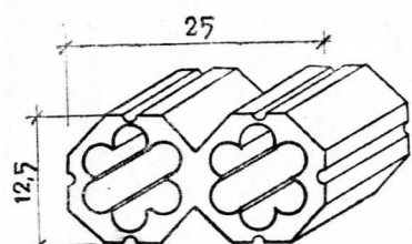
6. БЛОК АРХИТЕКТОРА ВЕРЖБИЦКОГО
