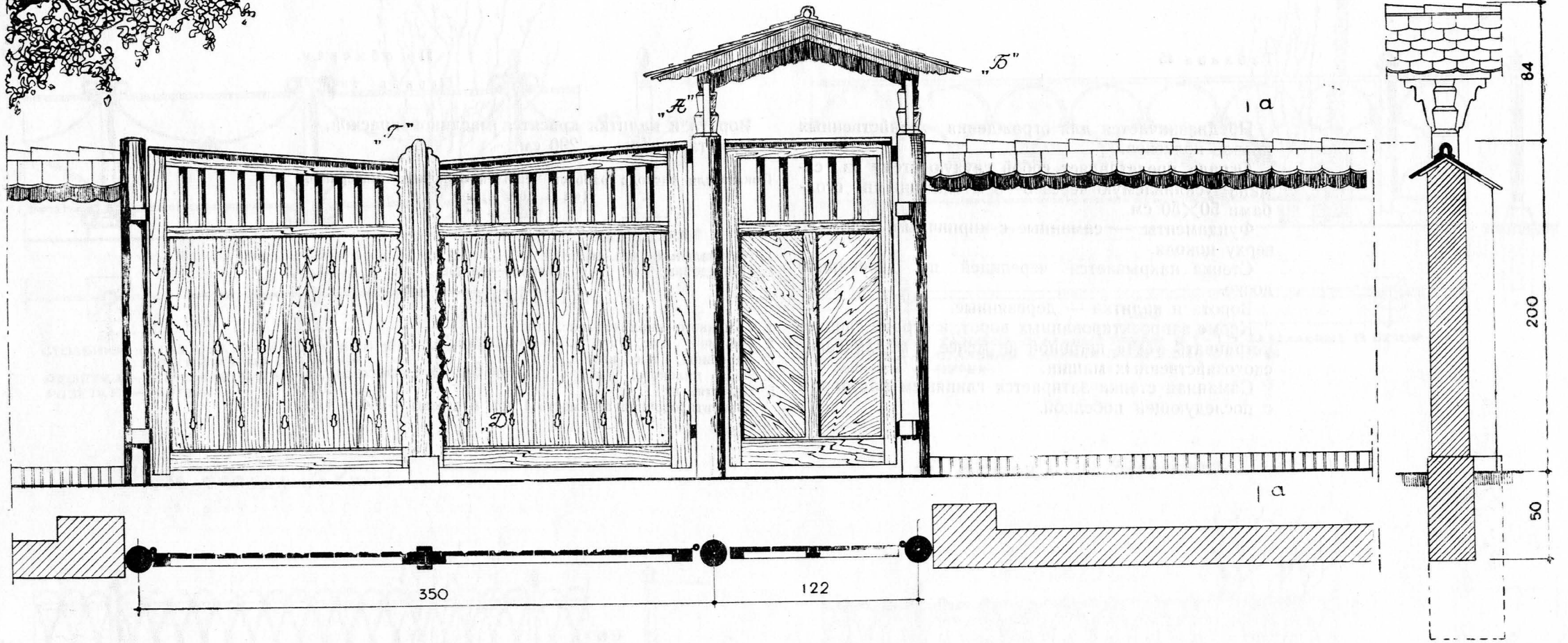
ДЕТАЛЬ "Д"
