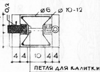
ДЕТАЛЬ А
