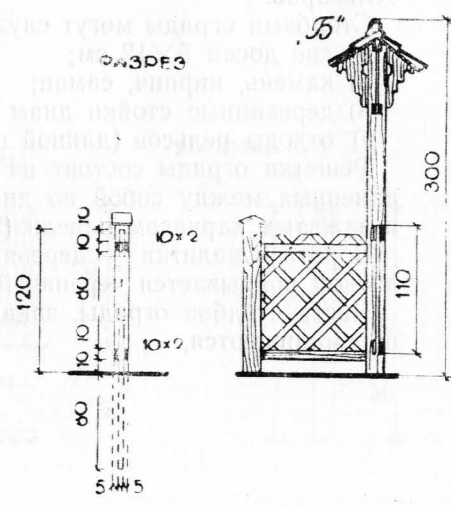
РАЗРЕЗ ПО ВХОДУ
