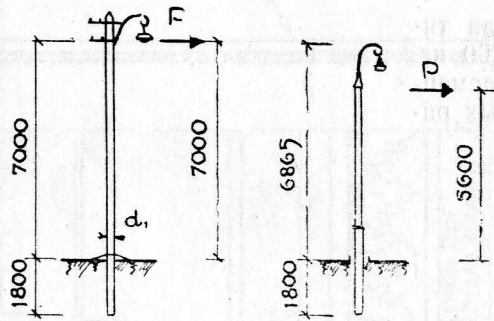
18. ОПОРА - СТОЛБ ИЗ ПОЛОСОВОЙ СТАЛИ
