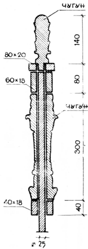
РАЗРЕЗ 1-1
