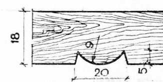
ПОРЕЗКА ДОСОК ЗАБОРА "Е"
