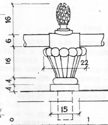
ДЕТАЛЬ "А"
