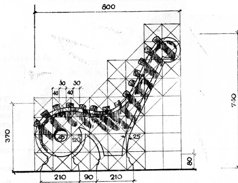
БОКОВОЙ ВИД
