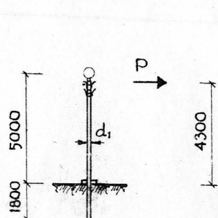
19. ОПОРА - СТАЛЬНАЯ ТРУБА
