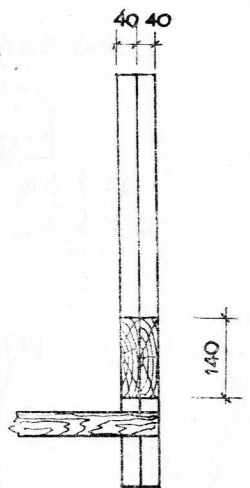
СЕЧЕНИЕ a-a
