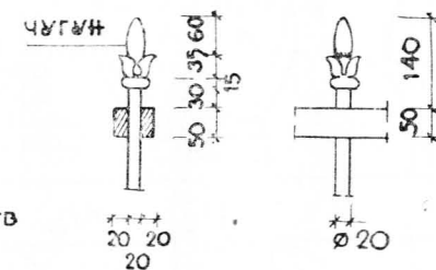
ДЕТАЛЬ "Д"
