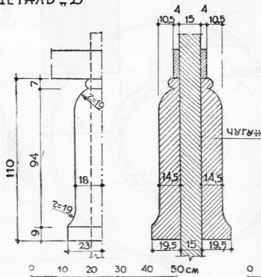
ДЕТАЛЬ „Д“
