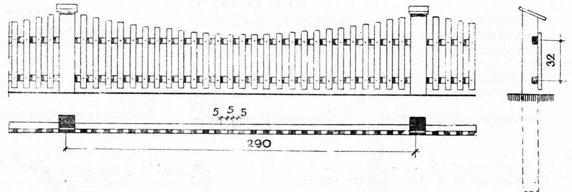
52. ДЕРЕВЯННАЯ ОГРАДА
