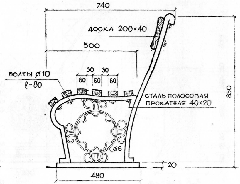
РАЗРЕЗ 1-1
