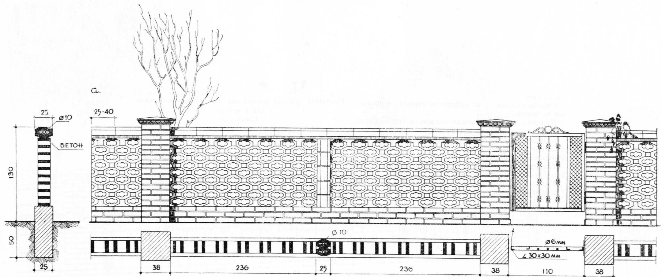
СХЕМА ОГРАДЫ
