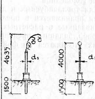
19. ОПОРА - СТАЛЬНАЯ ТРУБА
