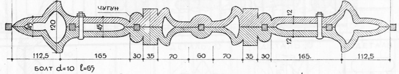
ДЕТАЛЬ „В“
