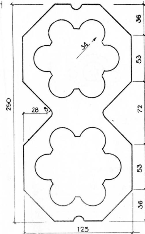
БЛОК ОГРАДЫ
