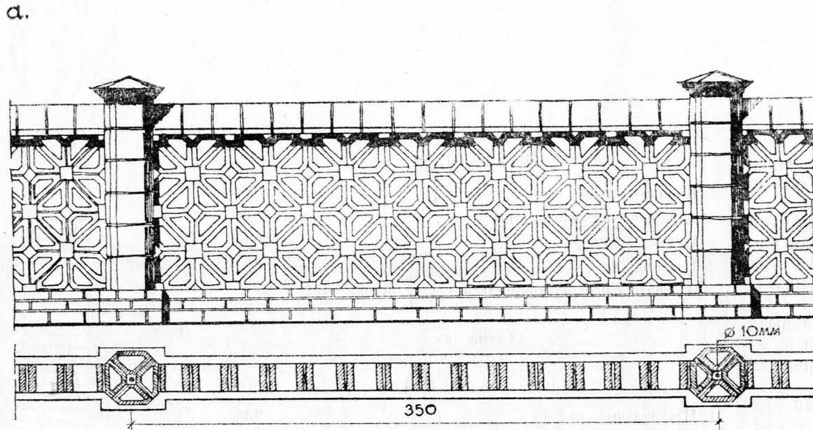
СХЕМА ОГРАДЫ
