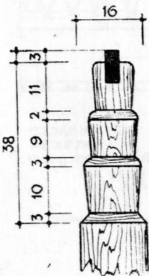
ДЕТАЛЬ "А"
