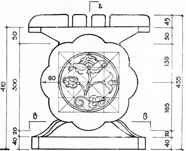
БОКОВОЙ ФАСАД ДЕТАЛЬ КЕРАМИЧЕСКОЙ ВСТАВКИ
