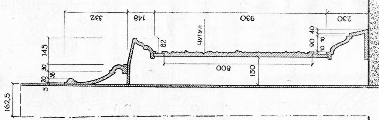
РАЗРЕЗ 5-5
