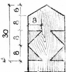
ВЕРХ СТОЛБИКА "Ж"
