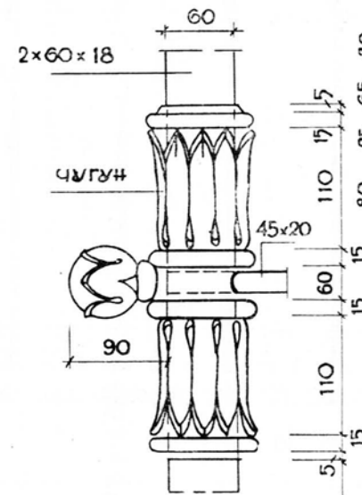
ДЕТАЛЬ „Ж“
