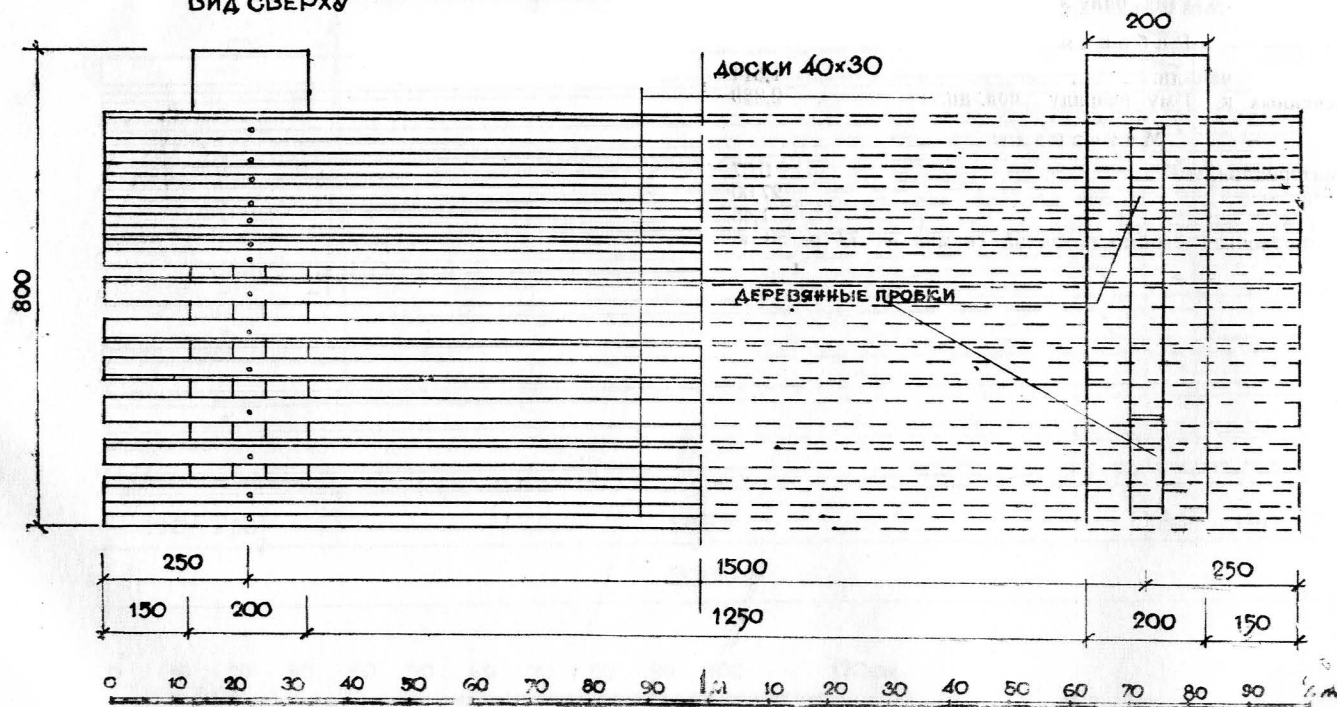
ВИД СВЕРХУ
