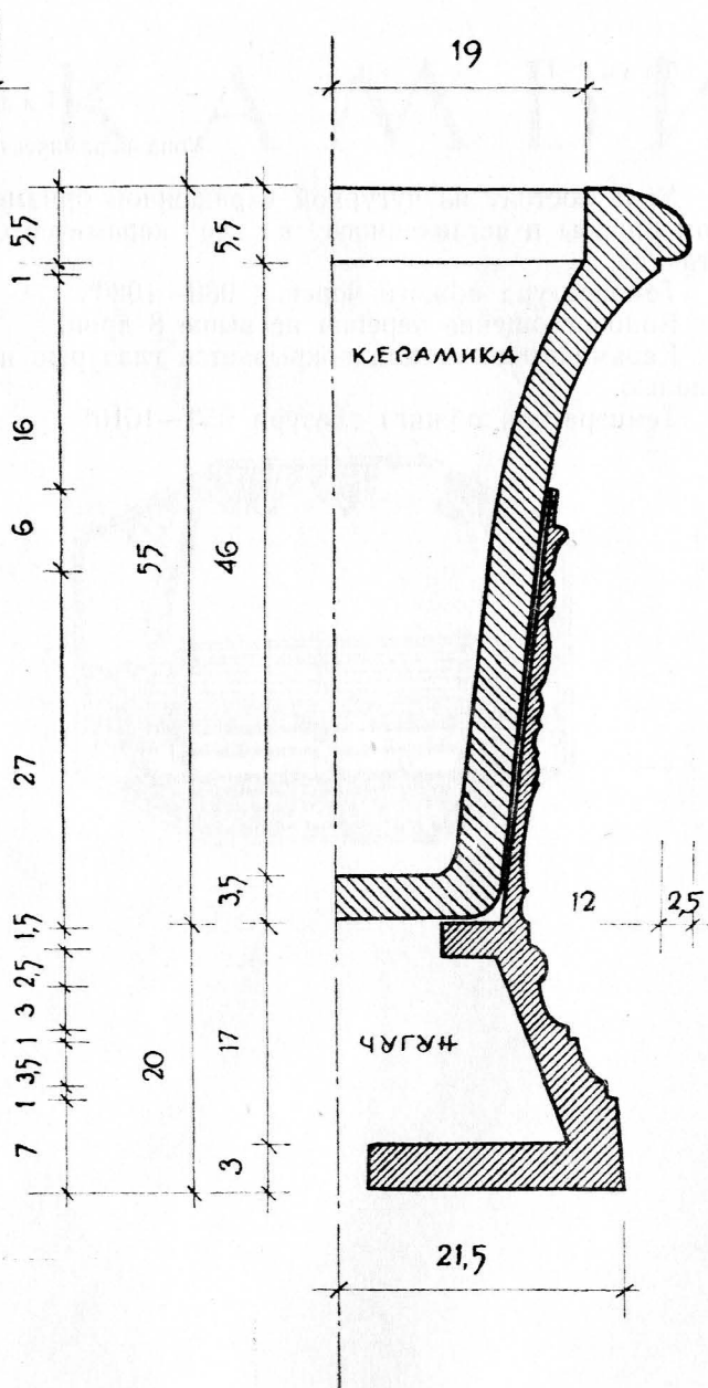
РАЗРЕЗ ПО ВЕРТИКАЛЬНОЙ ОСИ
