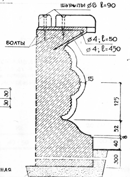
СЕЧЕНИЕ а-а
