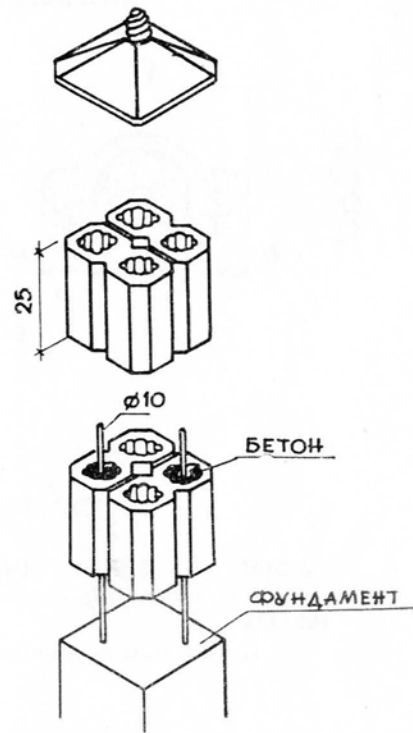
СХЕМА КЛАДКИ СТОЛБА
