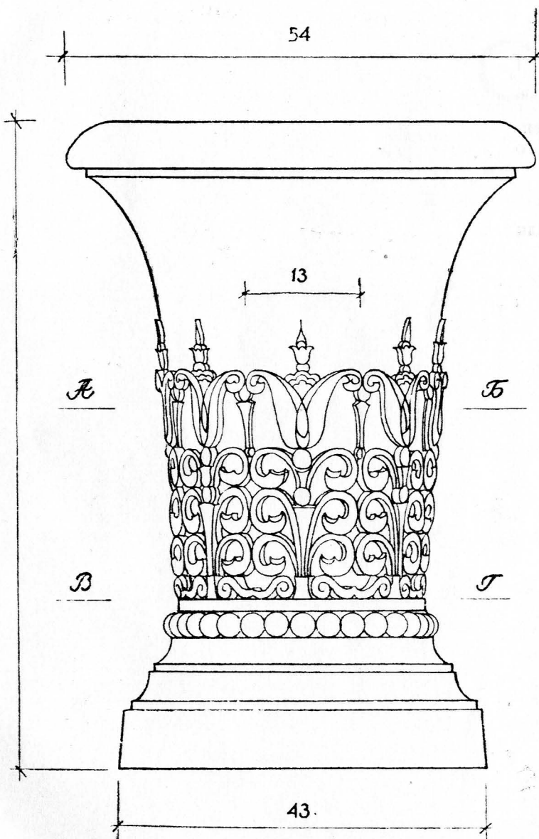
ОБЩИЙ ВИД УРНЫ
