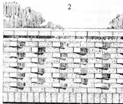
2 ГЛУХАЯ НАПУСК КИРПИЧА УГЛОМ
