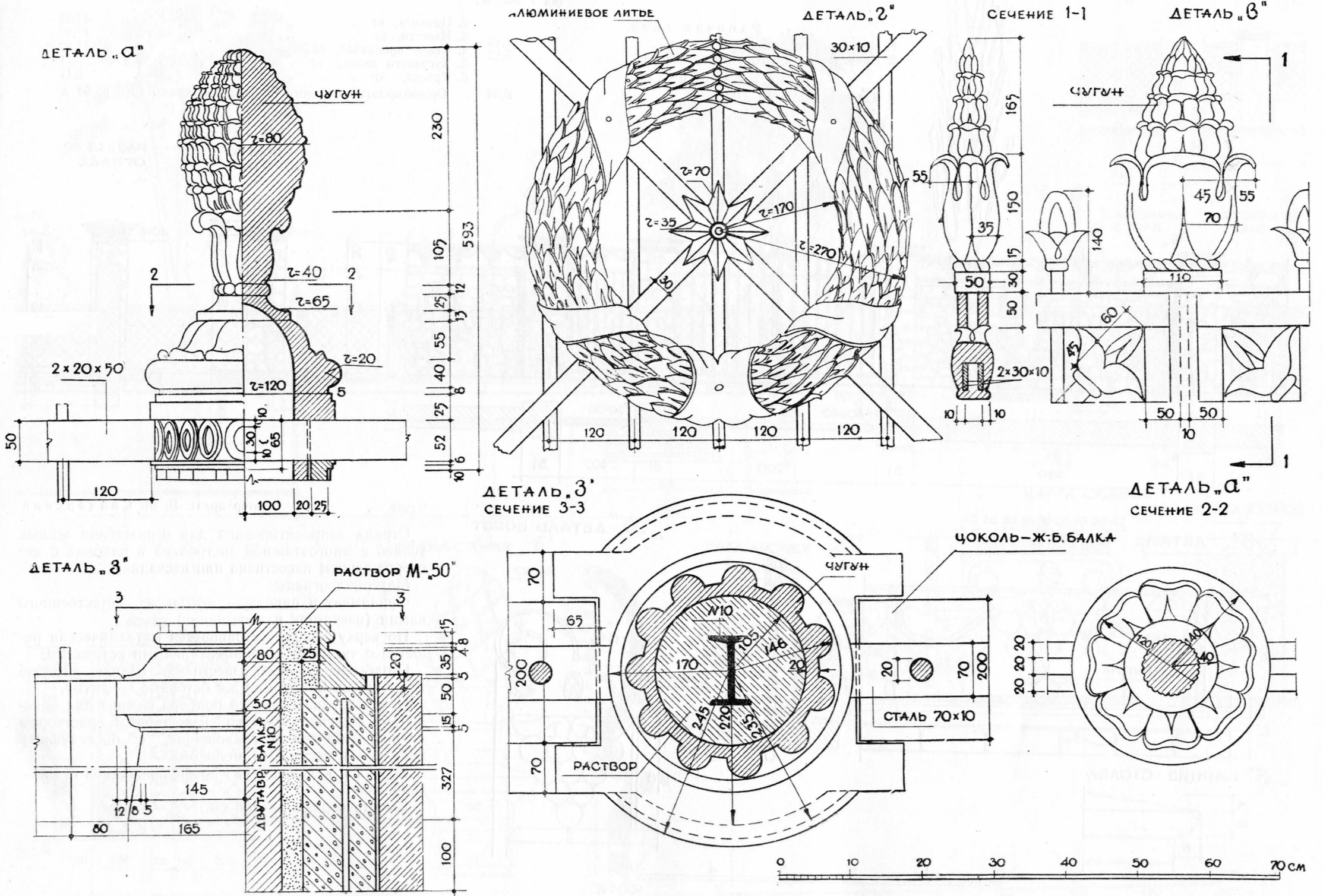
Детали к ограде тип 5
