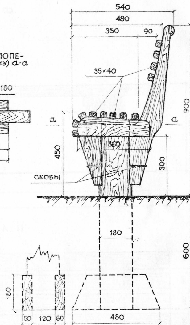
ВИД ПО 1-1
