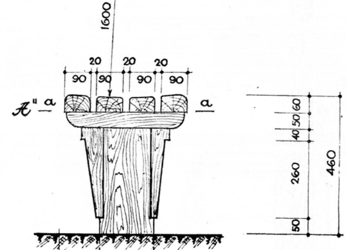
СЕЧЕНИЕ а-а
