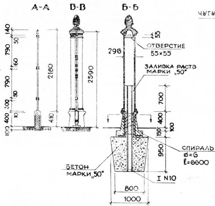
ДЕТАЛИ ОГРАДЫ - СМ ТАБЛИЦУ N 16
