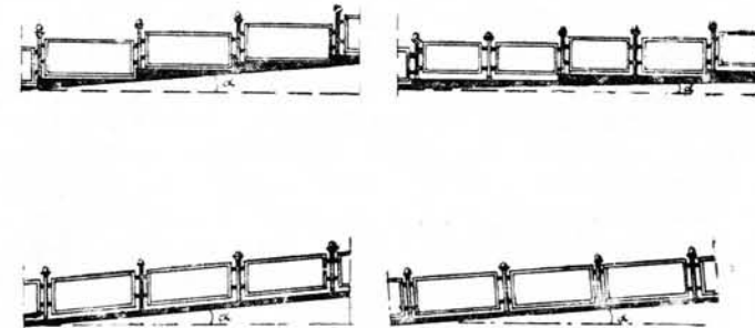
Рис. 12. Схемы оград на продольных уклонах улиц.
