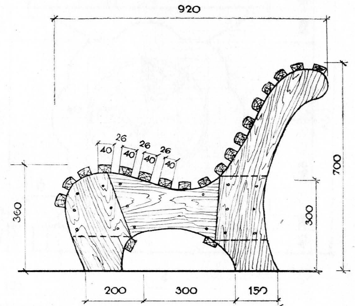
БОКОВОЙ ВИД
