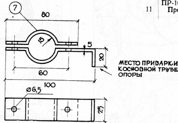
СКОБА ДЛЯ КРЕПЛЕНИЯ ВОРОНКИ
