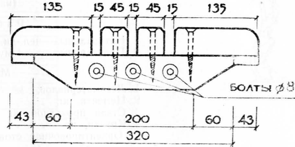
СЕЧЕНИЕ б-б
