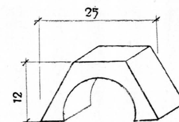
10. БЛОК АРХИТЕКТОРА СВИДЕРСКОГО
