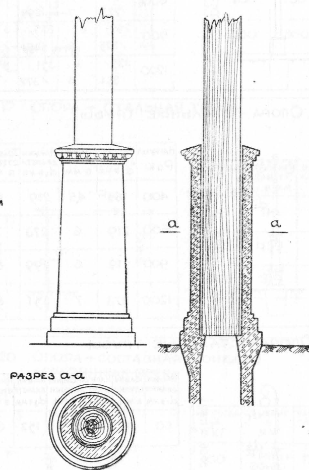
е ДЕРЕВЯННАЯ ОПОРА ЦОКОЛЬ-„ПАСЫНОК“-ЦЕНТРИ- ФУГИРОВАННЫЙ ЖЕЛЕЗОБЕТОН
