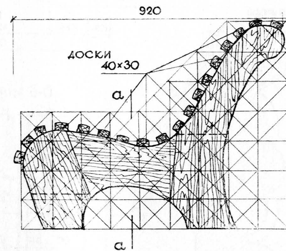
ДЕТАЛЬ Ж (ножка скамьи)
