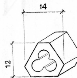
9. БЛОК АРХИТЕКТОРА ЛИБЕРБЕРГ
