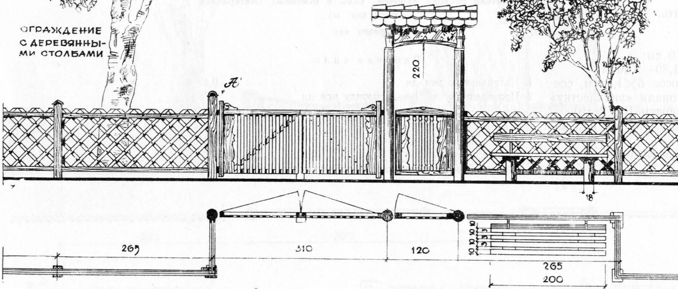
А ВОРОТА
