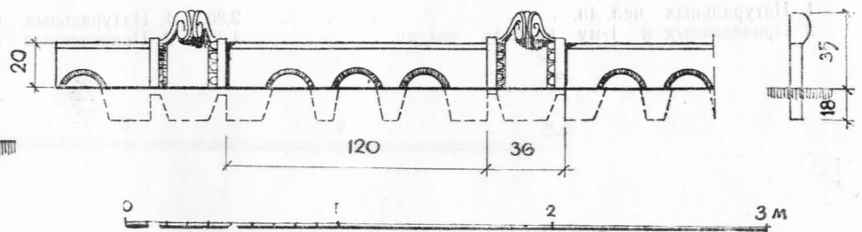
46. ОГРАДА ИЗ БЕТОННЫХ ПЛИТ
