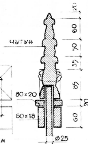
ДЕТАЛЬ „Ж“
