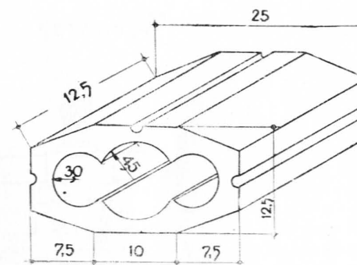
РАЗМЕРЫ БЛОКА ДАНЫ В ММ
